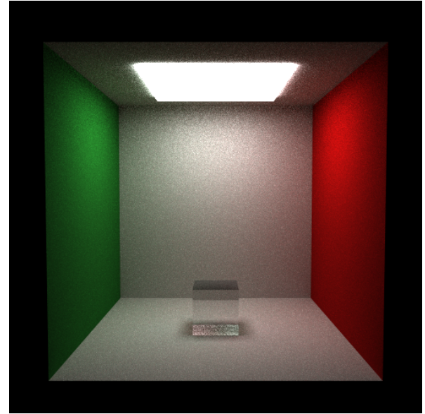
Figura 10. Água (IOR=1,33), absorção cromática, MIS sem RR (512×512, SPP=256, ≈142 min): convergência quase total, ruído praticamente eliminado.
