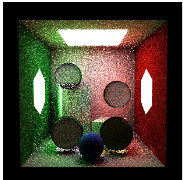
Figura 17. Cena combinada, mis (512×512, SPP=64, estratificado, depth=12 ): combina BSDF e NEE com heurística de potência ( \beta = 2 ); menor variância nas superfícies difusas e especulares; regiões TIR ainda visíveis nas bordas das esferas.
