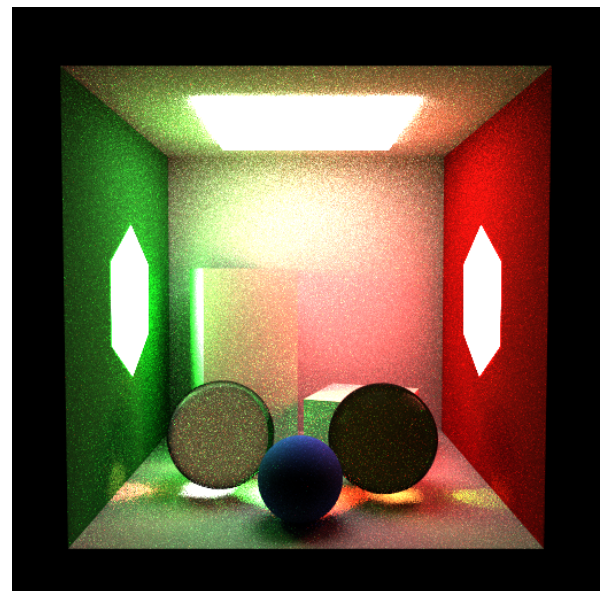
Figura 14. Showcase — mis + Roleta Russa (512×512, SPP=64, estratificado, depth=12, ≈70 min): mesma média, terminação probabilística de caminhos profundos.
