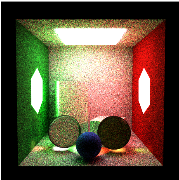
Figura 11. Showcase — bsdf_only (512×512, SPP=64, estratificado, depth=12, ≈42 min): alta variância; as fontes hexagonais laterais são raramente amostradas por BSDF puro.
