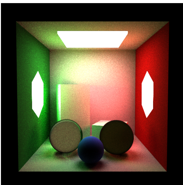
Figura 12. Showcase — nee_only (512×512, SPP=64, estratificado, depth=12, ≈100 min): amostragem direta das três fontes (teto + paredes laterais); iluminação direta nítida.
