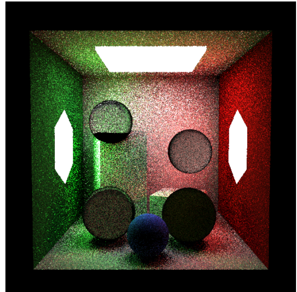
Figura 16. Cena combinada, nee_only (512×512, SPP=2, estratificado, depth=4 ): iluminação direta das três fontes nítidas nas superfícies difusas; esferas especulares ainda ruidosas pois NEE é pulado em bounces dielétricos ( is_specular ).
