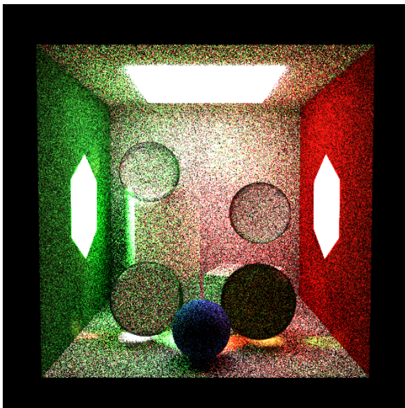
Figura 15. Cena combinada, bsdf_only (512×512, SPP=2, estratificado, depth=4 ): alta variância; esferas dielétricas com regiões escuras por depth esgotado e TIR.
