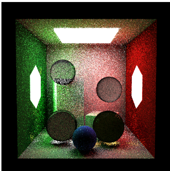
Figura 18. Cena combinada, mis + Roleta Russa (512×512, SPP=64, estratificado, depth=12): terminção probabilística de caminhos de baixo throughput ; reduz tempo de render mantendo estimador não-viesado.
