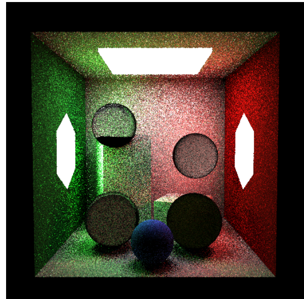
Figura 21. Cena combinada, nee_only (512×512, SPP=2, estratificado, depth=4): iluminação direta das três fontes nítida nas superfícies difusas; esferas especulares ainda ruidosas pois NEE é pulado em bounces dielétricos ( is_specular ).
