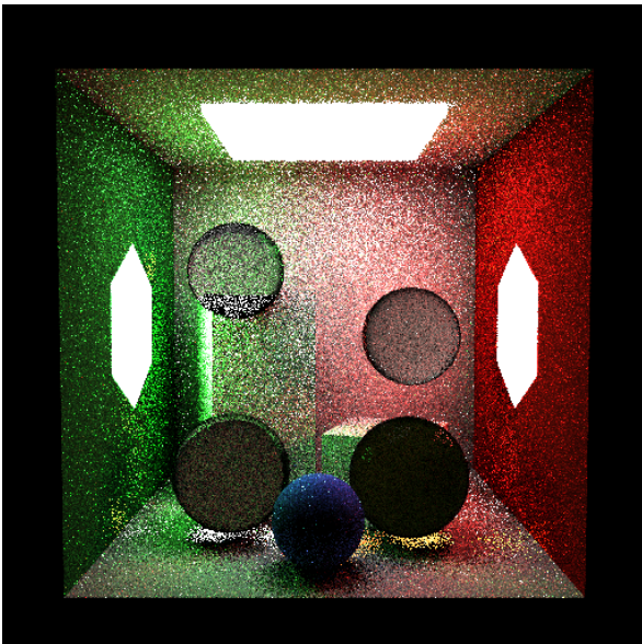
Figura 23. Cena combinada, mis + Roleta Russa (512×512, SPP=64, estratificado, depth=12): terminação probabilística de caminhos de baixo throughput; reduz tempo de render mantendo estimador não-viesado.
