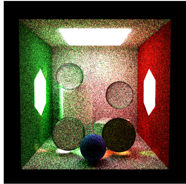
Figura 20. Cena combinada, bsdf_only (512×512, SPP=2, estratificado, depth=4): alta variância; esferas dielétricas com regiões escuras por depth esgotado e TIR.
