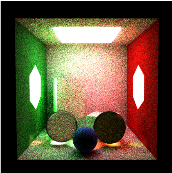
Figura 16. Showcase — bsdf_only ( 512 \times 512 , SPP=64 , estratificado, depth=12 , \approx 42 min): alta variância; as fontes hexagonais laterais são raramente amostradas por BSDF puro.
