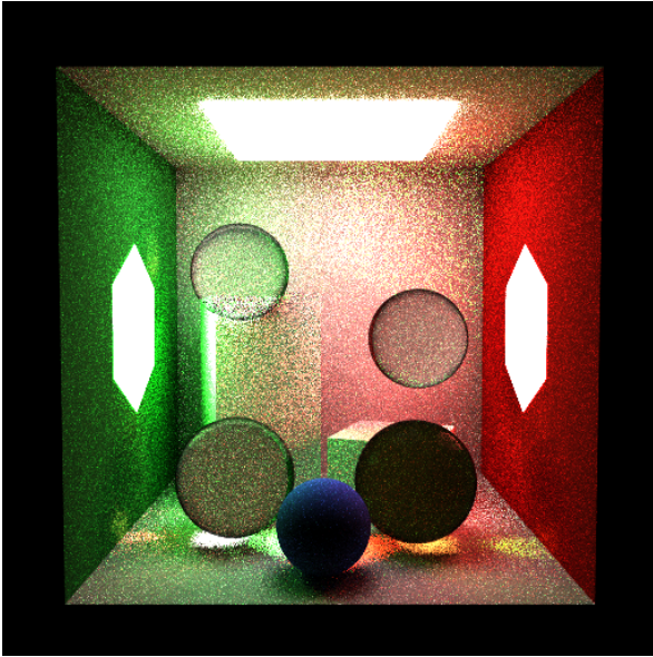
Figura 22. Cena combinada, mis (512×512, SPP=64, estratificado, depth=12): combina BSDF e NEE com heurística de potência ( \beta = 2 ); menor variância nas superfícies difusas e especulares; regiões TIR ainda visíveis nas bordas das esferas.
