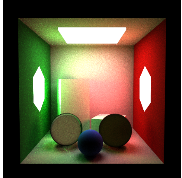
Figura 17. Showcase — nee_only ( 512 \times 512 , SPP=64 , estratificado, depth=12 , \approx 100 min): amostragem direta das três fontes (teto + paredes laterais); iluminação direta nítida.
