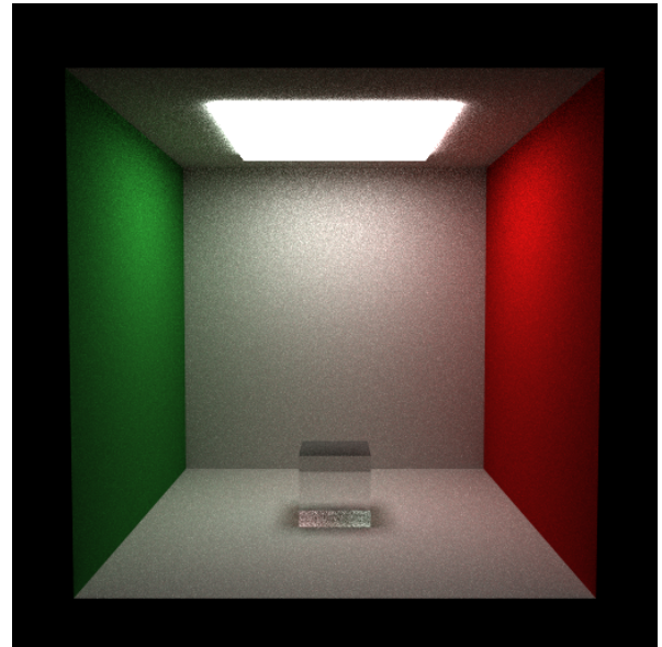
Figura 12. Água ( IOR=1,33 ), absorção cromática, MIS sem RR ( 512 \times 512 , SPP=256 , \approx 142 min): convergência quase total, ruído praticamente eliminado.
