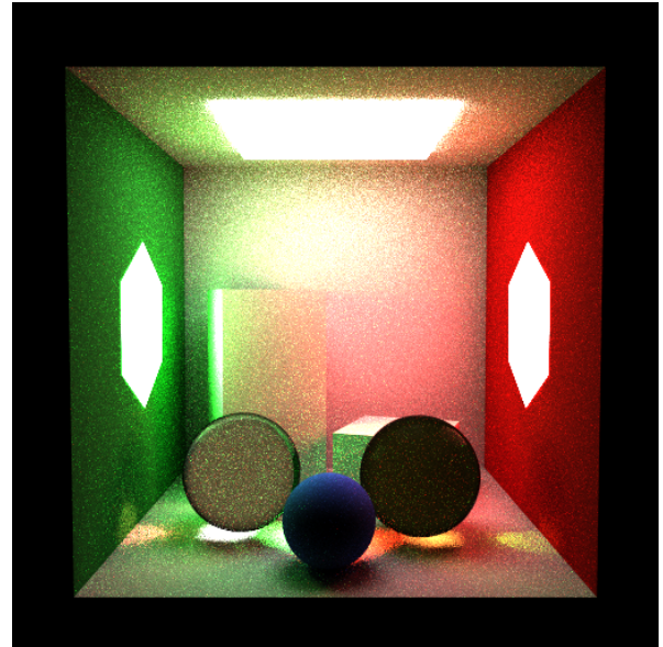
Figura 20. Wall lights — mis + Roleta Russa (512×512, SPP=64, estratificado, depth=12, ≈70 min): mesma média com terminação probabilística de caminhos profundos.
