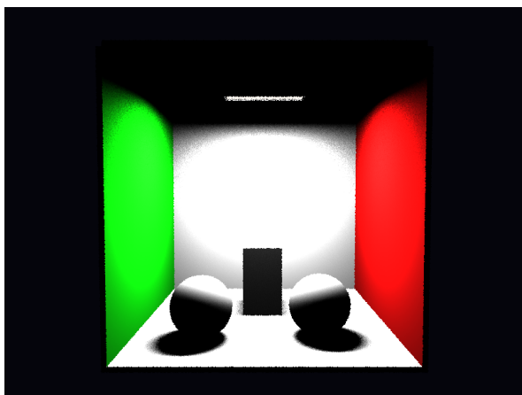
Figura 6. Cena com luz de área retangular e emissor visível: a penumbra vem da fonte extensa amostrada, enquanto a aparência luminosa do painel vem de EmissiveMaterial (800x600, spp=1).
