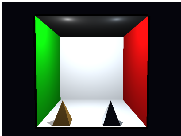
Figura 5. Cena triangular com BVH local: a imagem visualiza a malha sob o mesmo pipeline de iluminação, enquanto a poda por AABB reduz o custo interno da interseção (800x600, spp=1).
