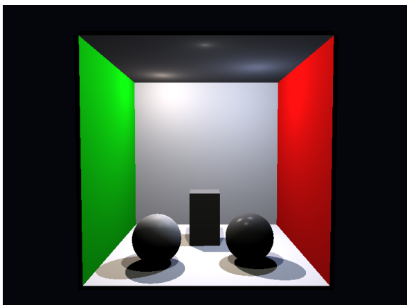
Figura 2. Cena com múltiplas luzes pontuais e variação do brilho especular em materiais com shininess distinto (800x600, spp=1).
