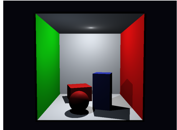
Figura 3. Cena de sombreado local com Phong e sombras diretas duras por visibilidade até a fonte (800x600, spp=1).
