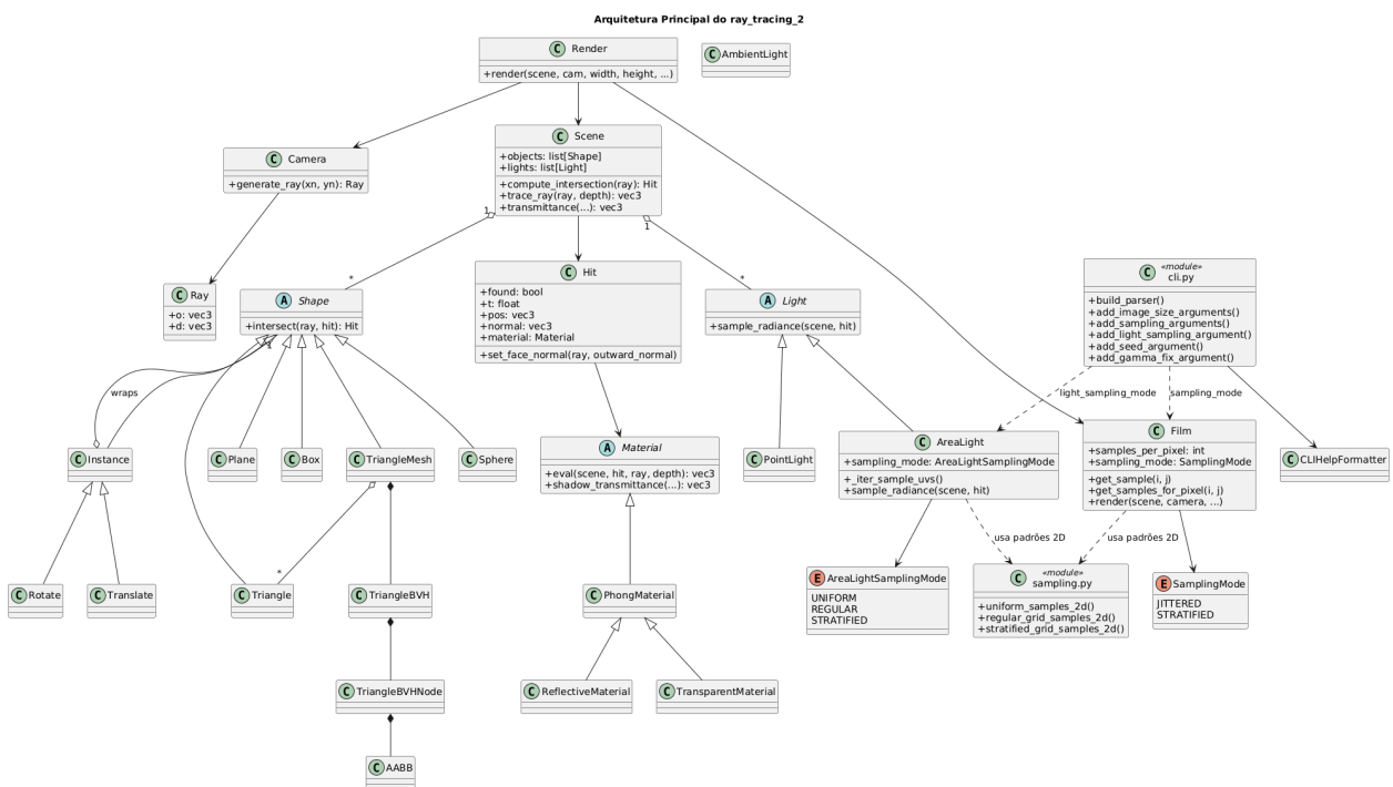
Figura 8. Diagrama de classes da arquitetura principal de ray_tracing_2.
