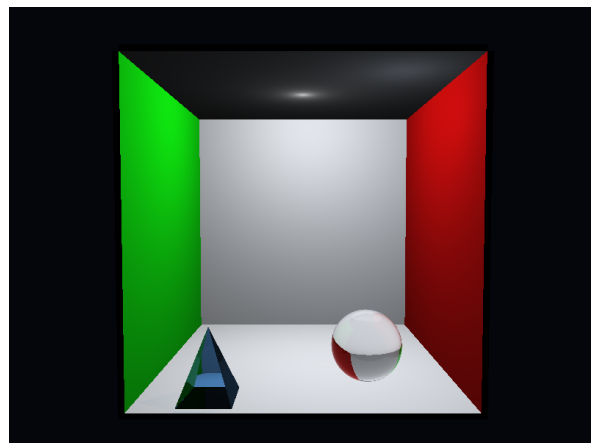
Figura 7. Cena com material refratário: o resultado combina Lei de Snell, reflexão interna total e atenuação tipo Beer-Lambert dentro do mesmo pipeline recursivo (800x600, spp=1).
