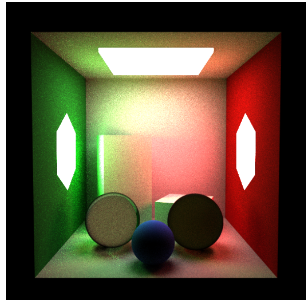
Figura 14. Showcase — nee_only (512×512, SPP=64, estratificado, depth=12, ≈100 min): amostragem direta das três fontes (teto + paredes laterais); iluminação direta nítida.
