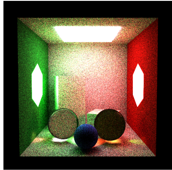
Figura 13. Showcase — bsdf_only (512×512, SPP=64, estratificado, depth=12, ≈42 min): alta variância; as fontes hexagonais laterais são raramente amostradas por BSDF puro.
