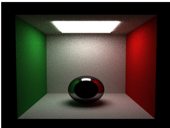
Figura 9. Esfera de vidro incolor (IOR=1,5), MIS sem RR (800×600, SPP=64, seed=42, ≈58 min). A alta reflectância Fresnel em ângulos rasantes — comportamento correto de DielectricBSDF \delta amostrado estocasticamente — confere aparência especular às bordas; refração e TIR são observáveis na região central da esfera.
