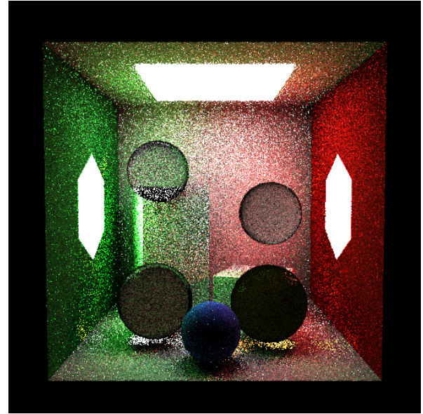
Figura 20. Cena combinada, mis (512×512, SPP=64, estratificado, depth=12): combina BSDF e NEE com heurística de potência ( \beta = 2 ); menor variância nas superfícies difusas e especulares; regiões TIR ainda visíveis nas bordas das esferas.
