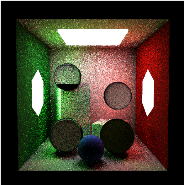
Figura 19. Cena combinada, nee_only (512×512, SPP=2, estratificado, depth=4): iluminação direta das três fontes nítida nas superfícies difusas; esferas especulares ainda ruidosas pois NEE é pulado em bounces dielétricos ( is_specular ).
