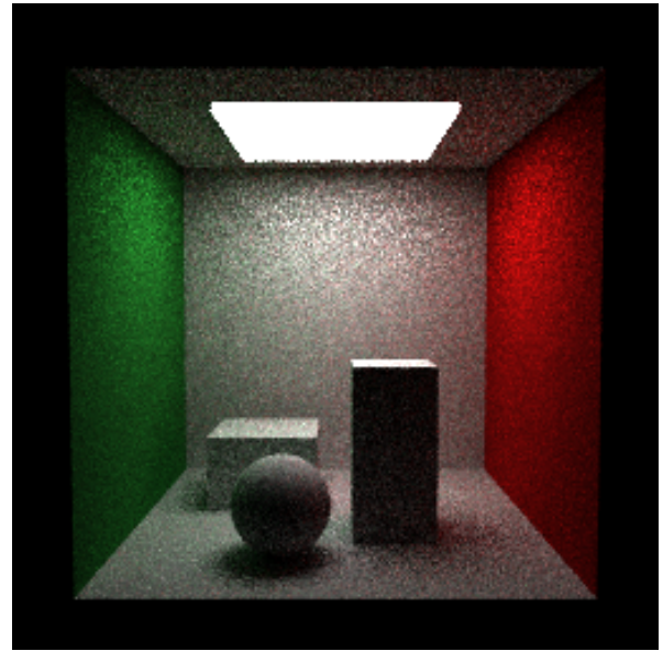
Figura 2. NEE — execução 1 ( 256 \times 256 , SPP=16, seed=42, \approx 1.89 min): amostragem direta da luz, menor variância que BSDF-only.
