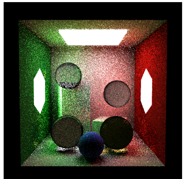
Figura 21. Cena combinada, mis + Roleta Russa (512×512, SPP=64, estratificado, depth=12): terminação probabilística de caminhos de baixo throughput ; reduz tempo de render mantendo estimador não-viesado.
