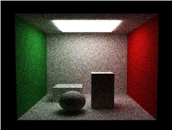
Figura 1. Cornell Box difusa, amostragem por BSDF ( 800 \times 600 , SPP=32, seed=42).
