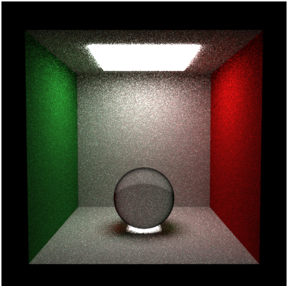
Figura 9. Esfera de vidro incolor (DielectricBSDF, IOR=1,5), MIS sem RR (512×512, SPP=32, ≈16 min): transparência com refração de Snell visível na região central; reflexão Fresnel nas bordas em ângulos rasantes; padrão de cáusticas no piso.
