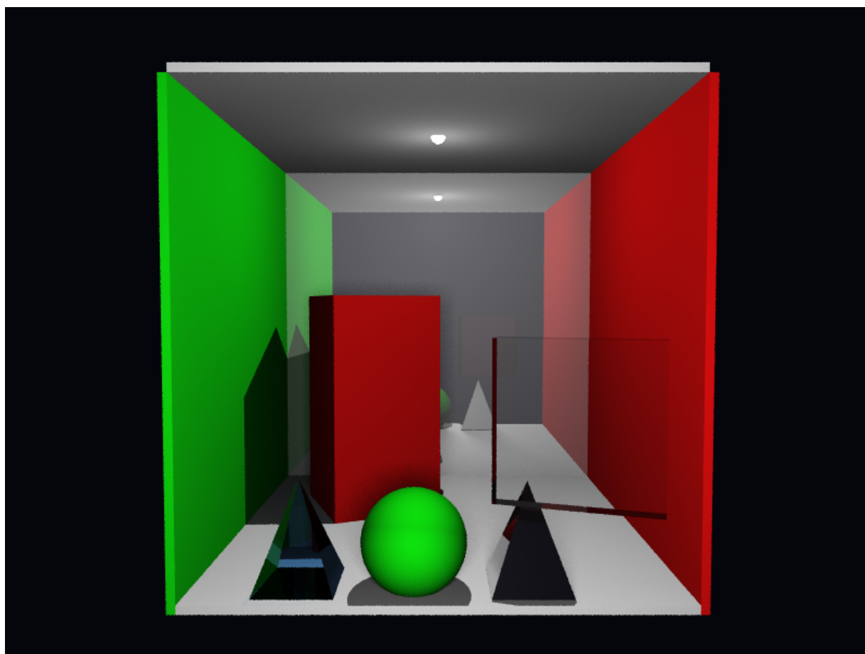
Figura 38. Variação adicional de cornell_box_pyramid : 10 amostras em jittered , malhas triangulares e luz de área estratificada.
