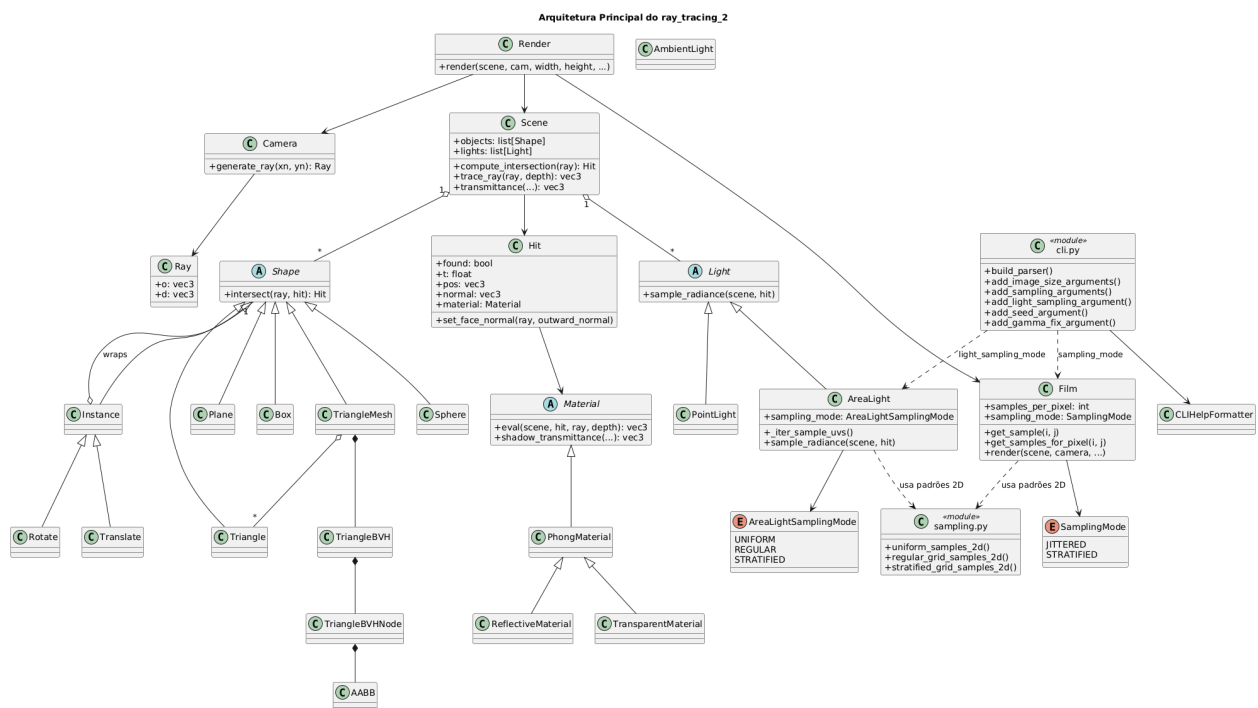
Figura 16. Diagrama de classes da arquitetura principal de ray_tracing_2.
