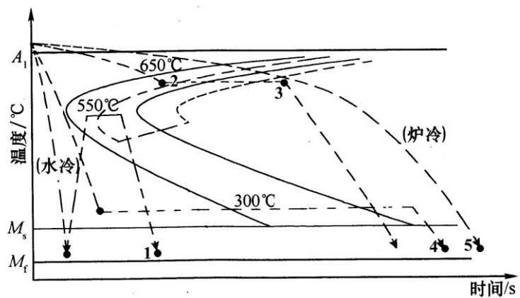
图 1 共析钢的 C 曲线和冷却曲线
