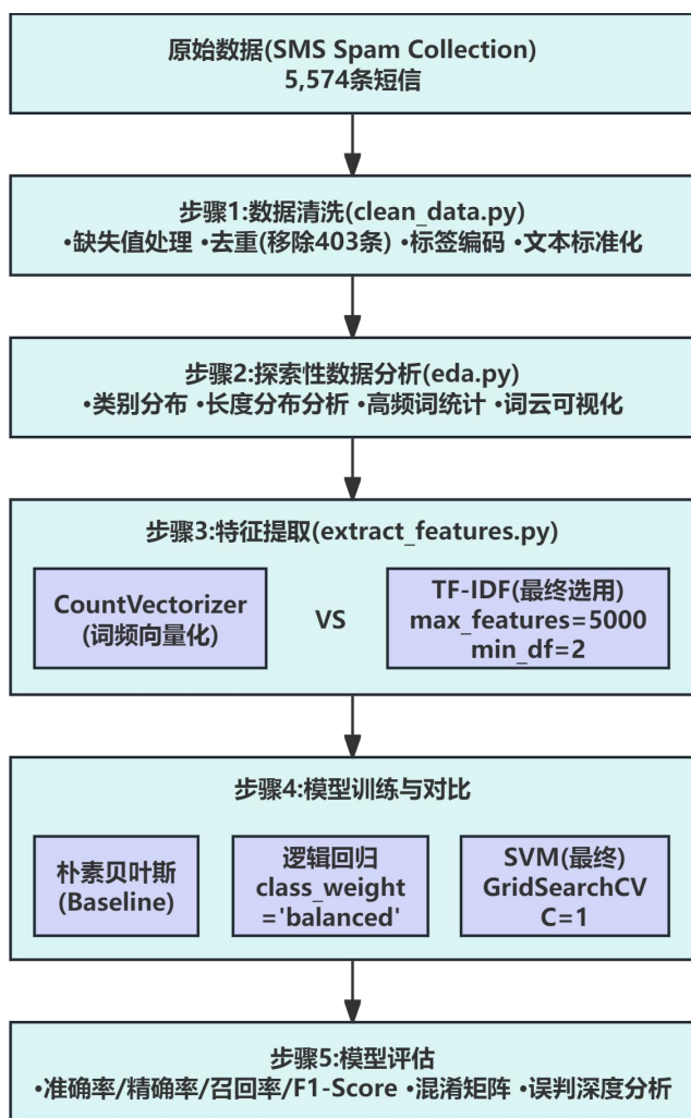
图5 垃圾短信检测方法流程图
