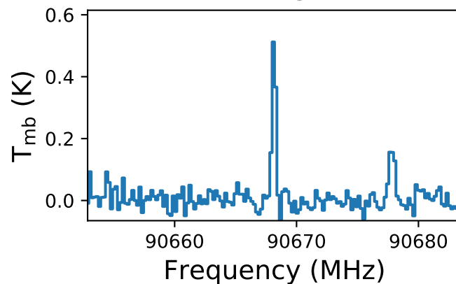
HNC
