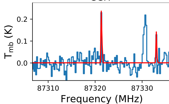
HNC
