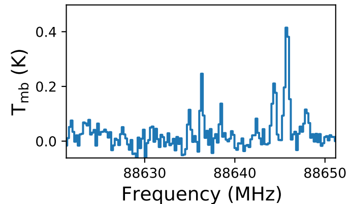
HCN
