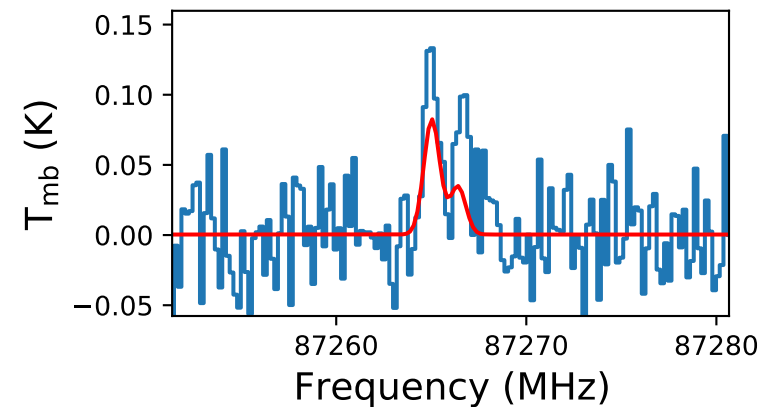
CCH
