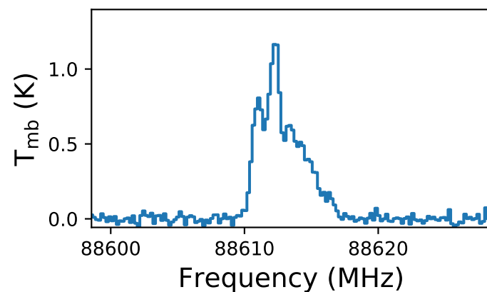
HCN
