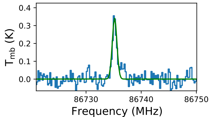
CCH
