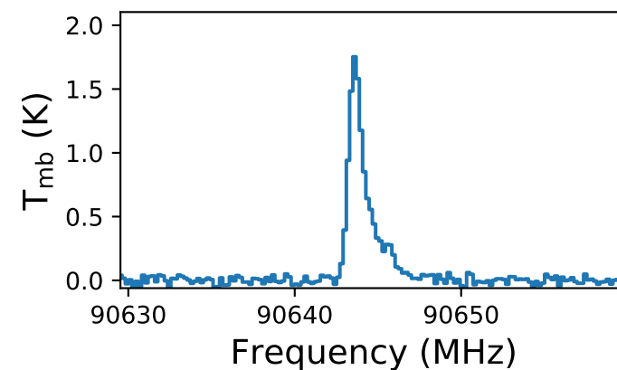
HNC
