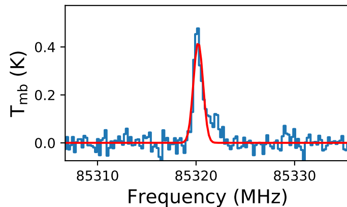
CCH
