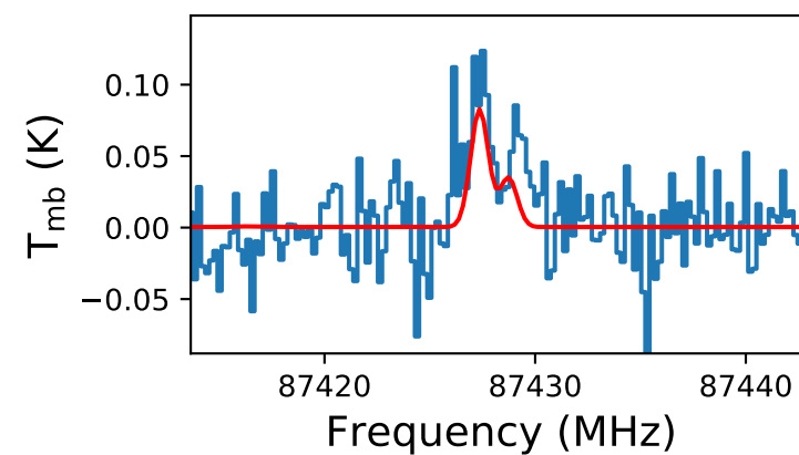
HNC
