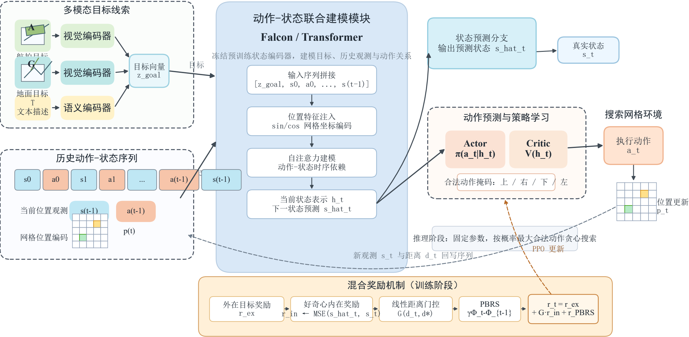
基于好奇心驱动的无人机主动目标定位导航总体结构
