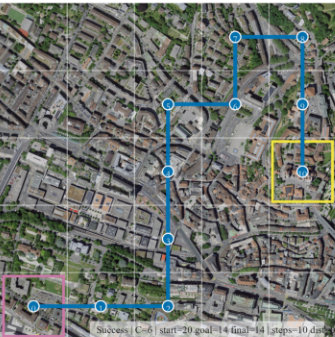
Ours
