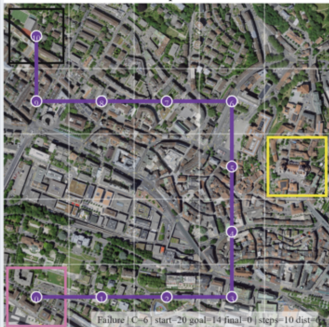
GeoExplorer
