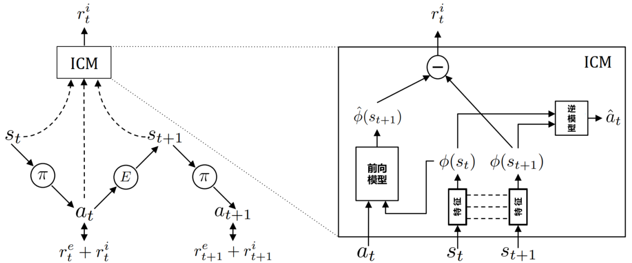
图 3 ICM 框架图 [32]
