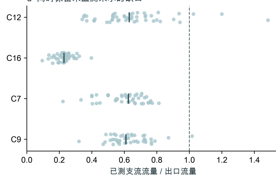
d 同时保留未监测来水的缺口
