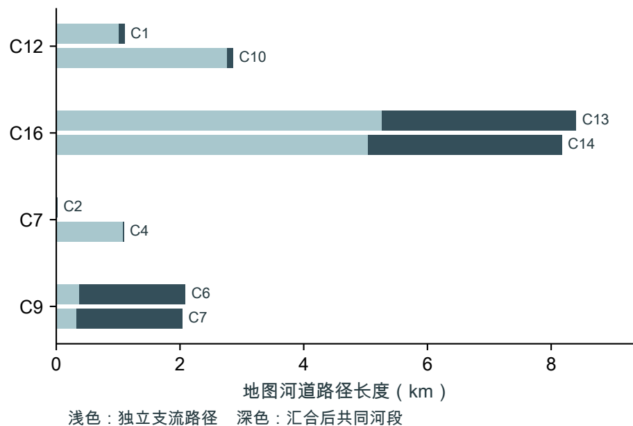
a 支流路径与共同下游河段
