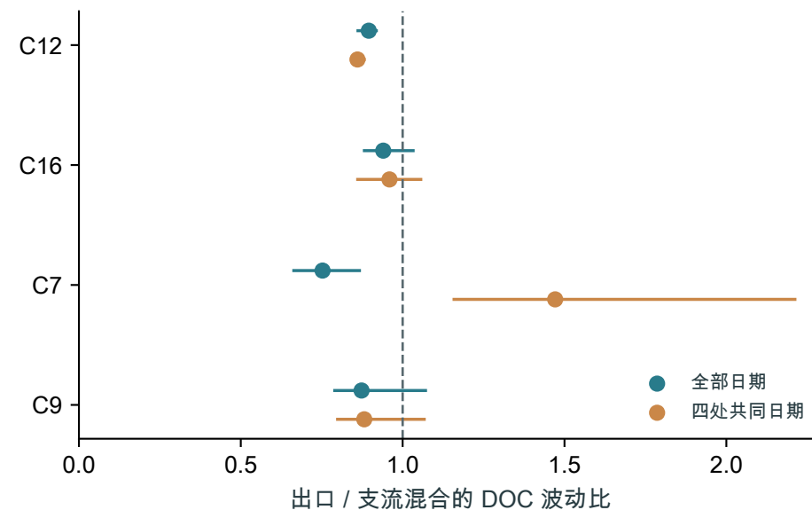
b 去除季节与年份趋势后的波动
