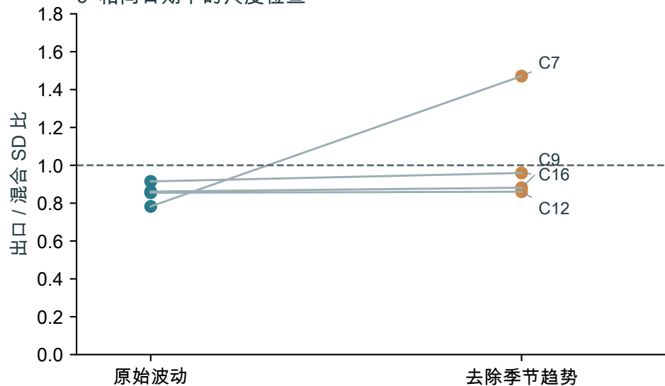
c 相同日期下的尺度检查
