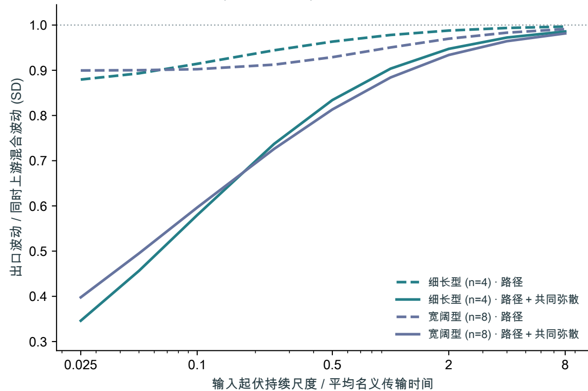
c 同输入下的形态比较 ( 覆盖 \geq 80\% )
