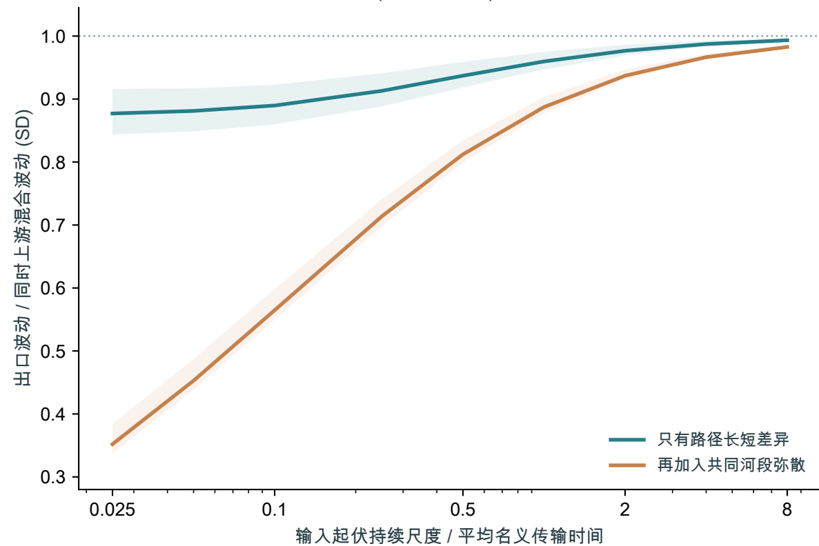
a 短促与缓慢变化的响应不同 ( 32个河网 )
