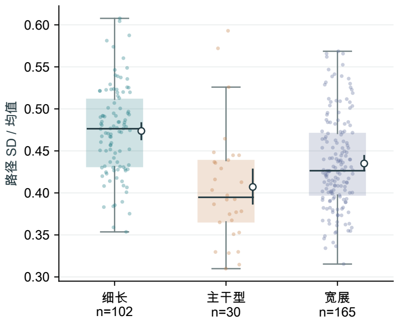
a 全河网到达分散
