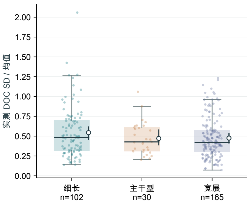
e 实测月度 DOC 波动
