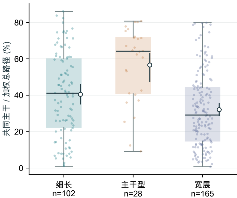
b 主要汇流后的共同路径
