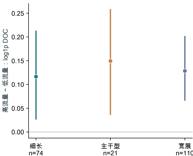
f 季节 / 年份调整后的响应
