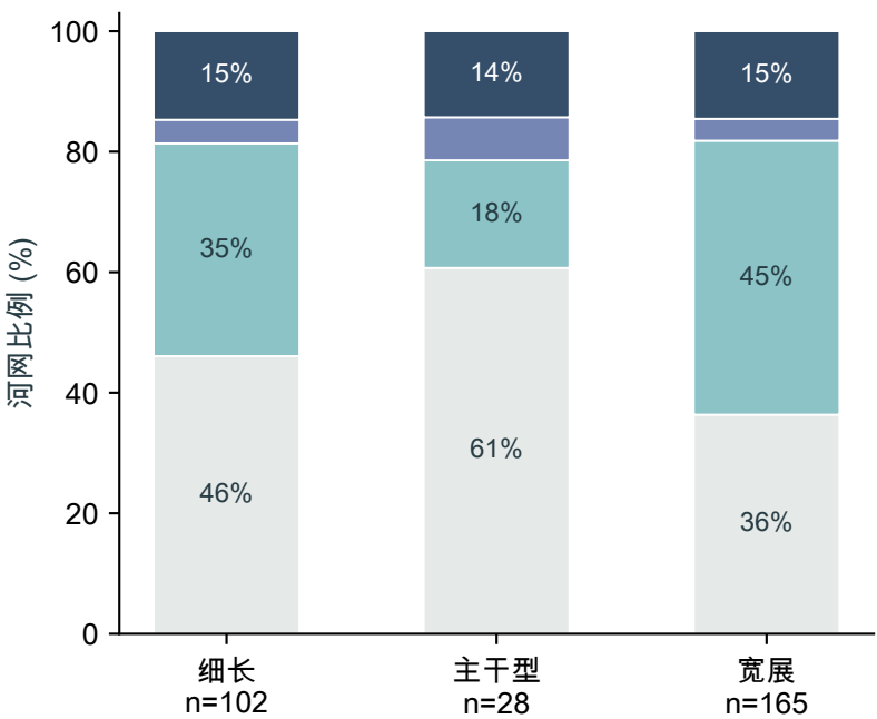
c 真实湖库位于哪段路径？
