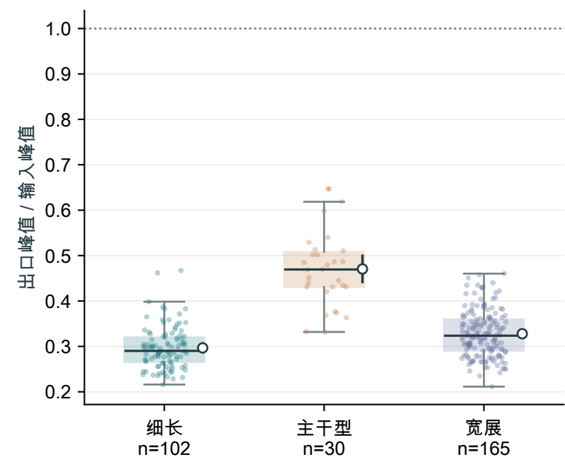
d 相同输入下的结构响应
