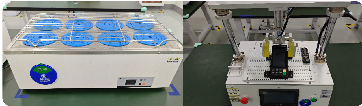
商米製造工廠實驗室設備（油炸實驗（左），底座壽命試驗（右））
