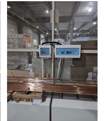
整改后：改造电路做到一机一闸
