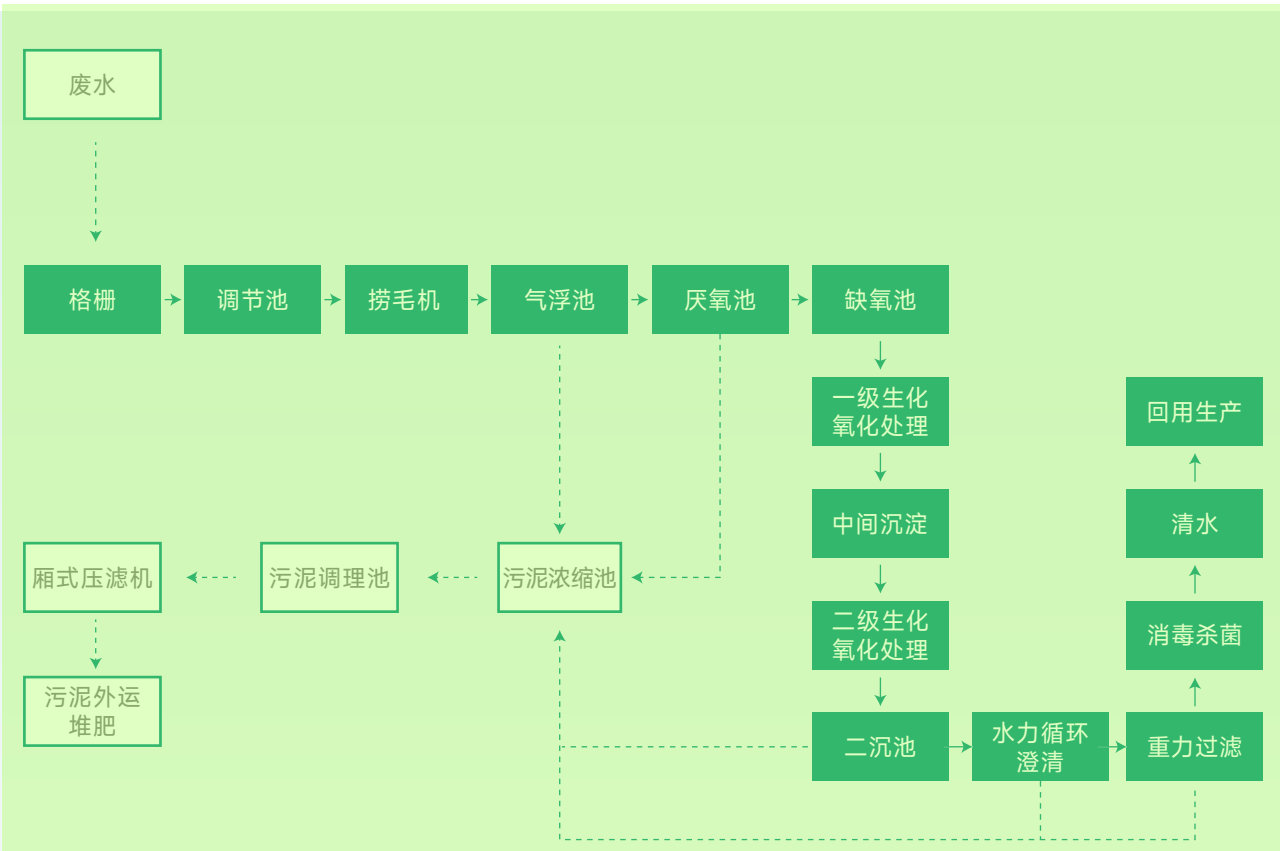
中水回用工艺流程示意图
