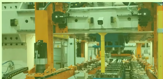
底壳伺服冲压线 15
