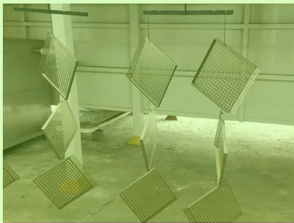
改善后的涂挂装工艺 15
