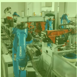
燃热面壳铆接线 19
