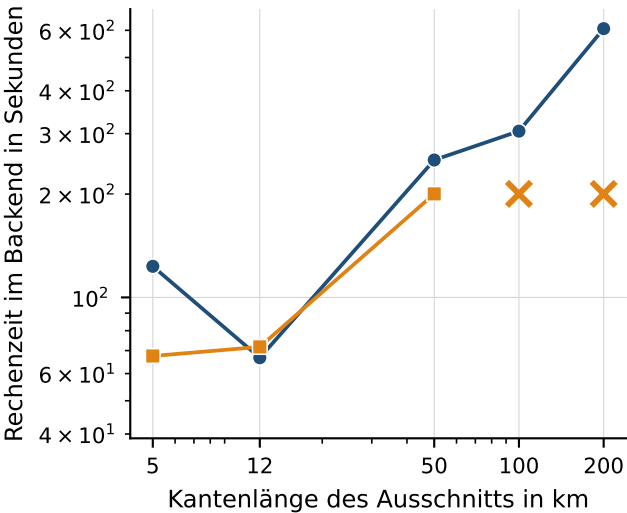
CDSE
