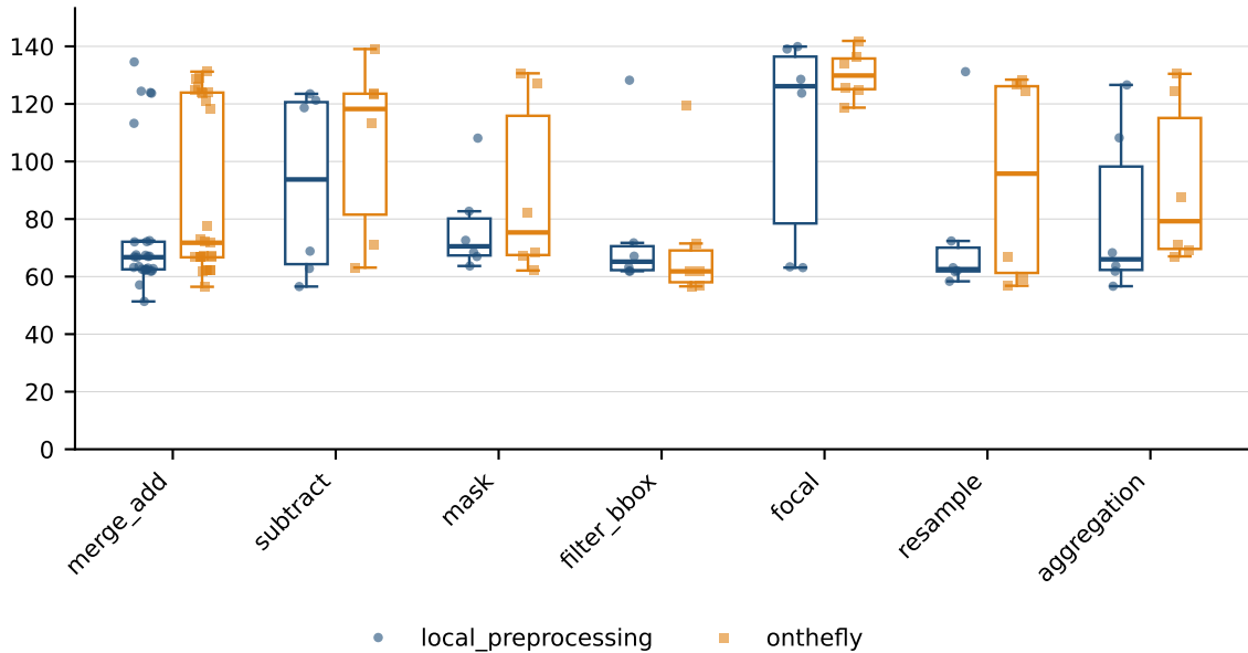
Rechenzeit im Backend in Sekunden
