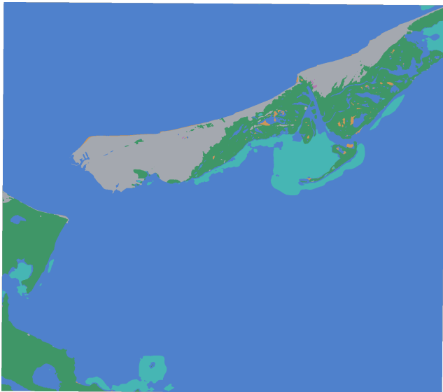
Mapa de hábitats
