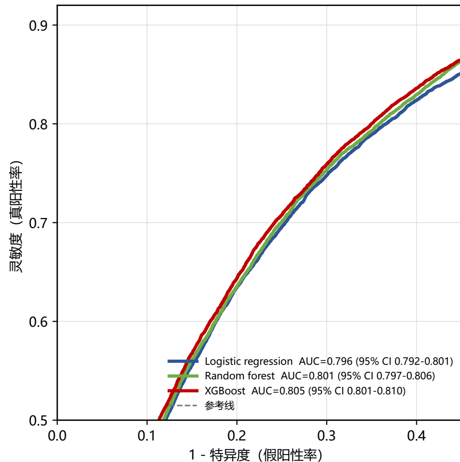
机器学习算法的3折交叉验证ROC曲线（局部放大）
