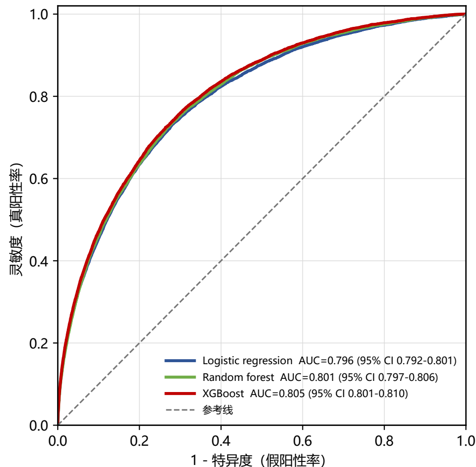
机器学习算法的3折交叉验证模型ROC曲线
