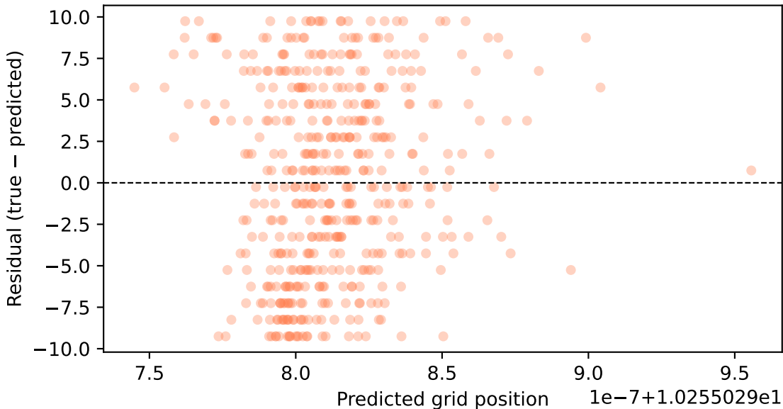
SVR_weather_only: Residual Plot
