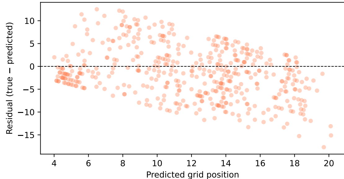
MLP_no_weather_no_fp: Residual Plot
