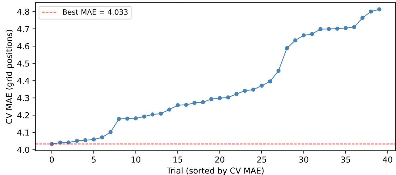
MLP_no_weather_no_fp: Hyperparameter Search Results
