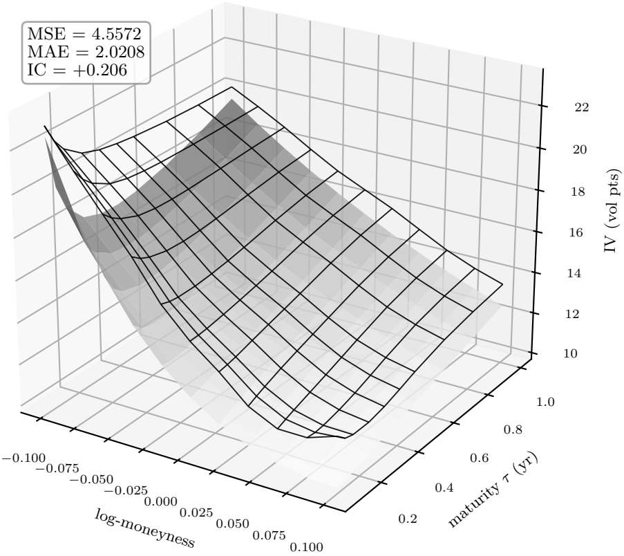
VAR
