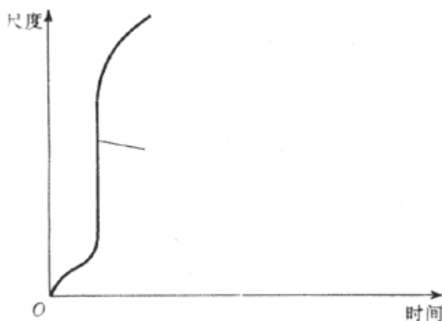
图 3-3 暴胀演化图象 按这个理论，宇宙在大爆炸中起源后不久，它的尺度便突然增大。图中的垂直方向比例已被大大缩小。暴胀相之后，膨胀速度不断减小，其变化方式与图 3-2 所示的情况非常相似。
