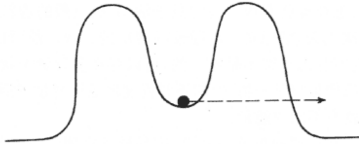
图 10-2 隧道效应 如果粒子陷入两座小山间的谷地中,它有很小的概率能通过借贷能量越过小山逃出去。实际上,这是在观察穿越势垒的隧道效应。一种熟悉的情况是某些元素原子核中的 \alpha 粒子通过隧道效应穿越核力势垒并飞离原子核,这种现象称为 \alpha 放射性。在这个例子中,“小山”由核力及电力产生,这里画的只是示意图。
