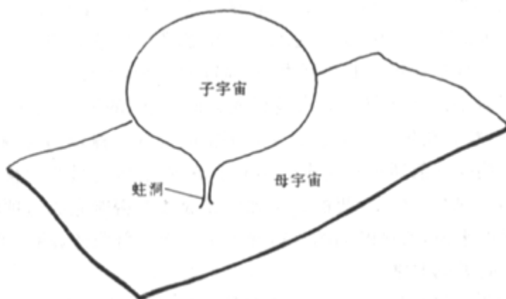
图 10-4 一个空间气泡像气球那样从母宇宙中长地来，这就形成了一个子宇宙，它通过脐带蛀洞与母体相连。从母宇宙的角度来看，蛀洞的嘴犹如一个黑洞。随着这个黑洞的蒸发，蛀洞的咽喉就掐断了，因此同母宇宙失却了联系。接着婴宇宙凭借自己的地位成为一个独立存在的宇宙。
