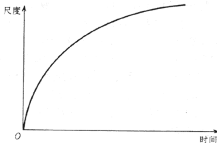
图 3-2 宇宙膨胀速度大致按图示的方式随时间逐步减小。在这个简单模型中，时间轴上标上 0 的那一点的膨胀速度为无限大，它对应着大爆炸。
