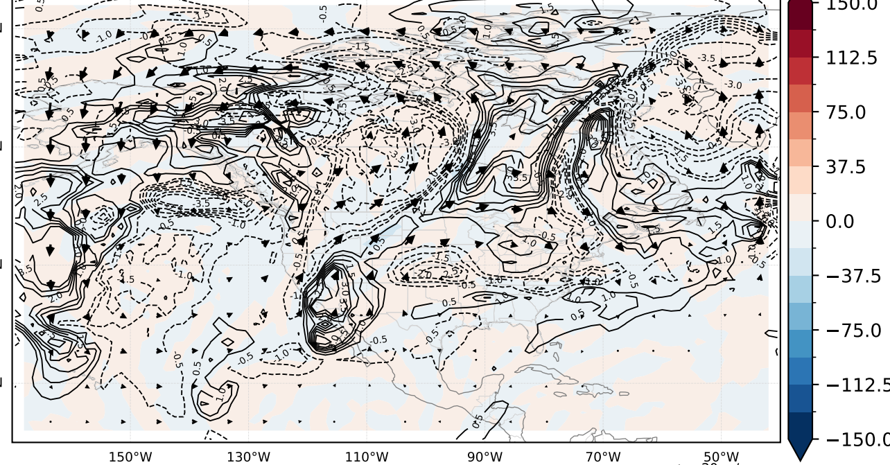
(d) Lower piece: 1000-850 hPa
