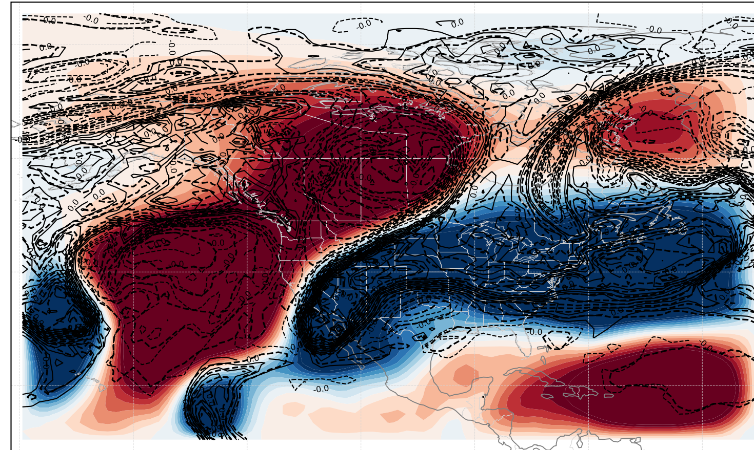
Upper (300-200 hPa)
