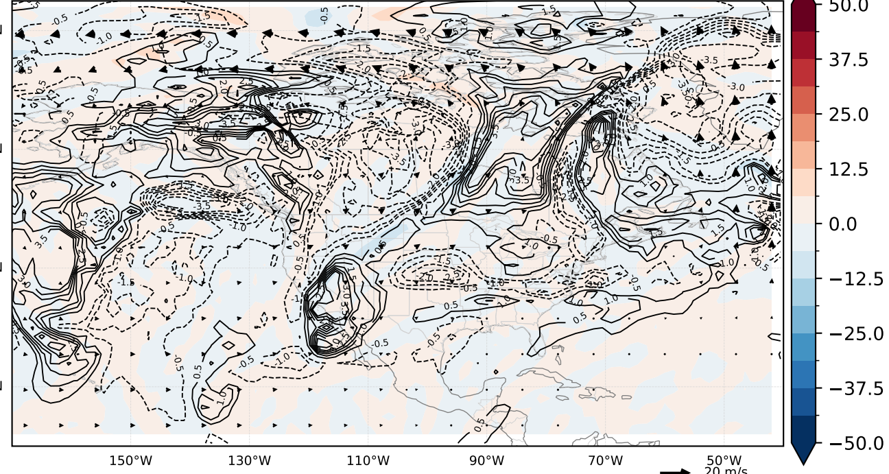
(d) Lower piece: 1000-850 hPa
