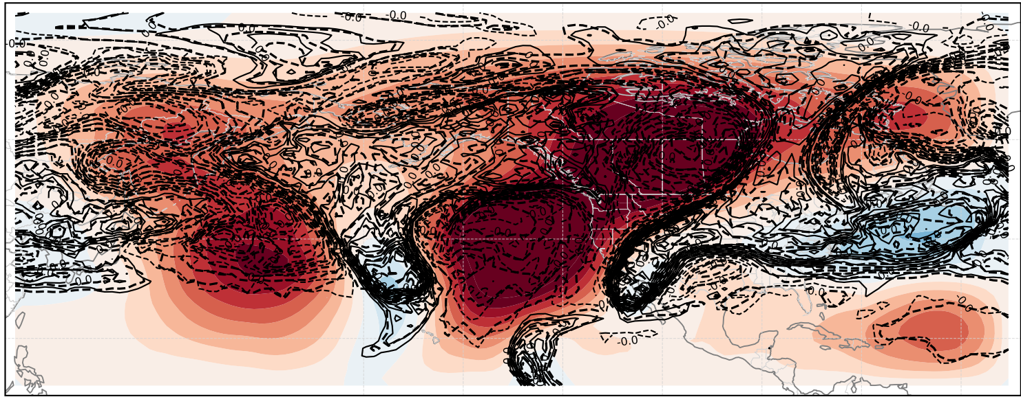
Upper (300-200 hPa)
