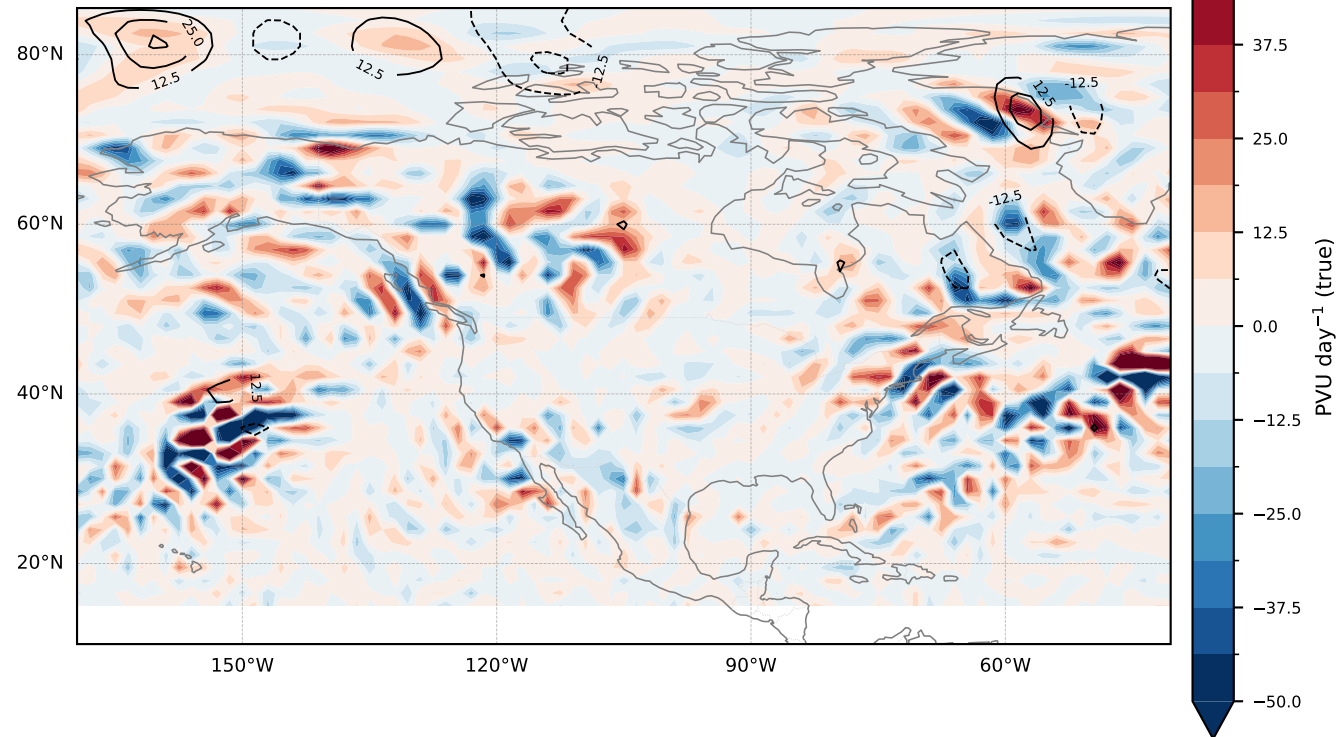
(d) Sum vs. true tendency (shade=true, contour= \Sigma pieces)
