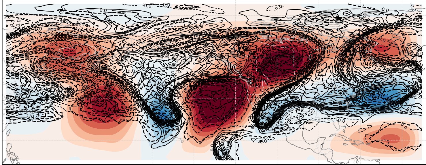
Upper (400-200 + 100 (θ) hPa)
