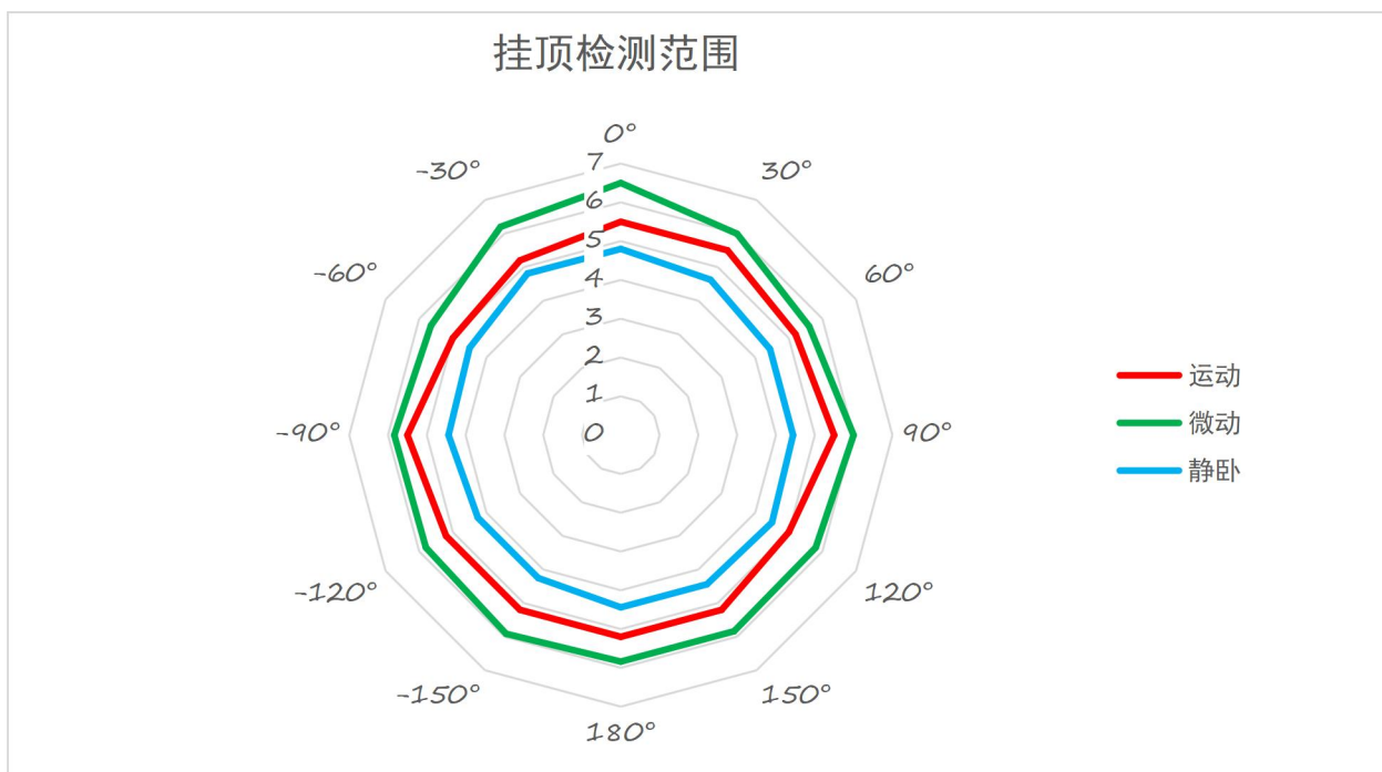
图 6-4 HLK-LD2402-L 挂顶安装感应范围
