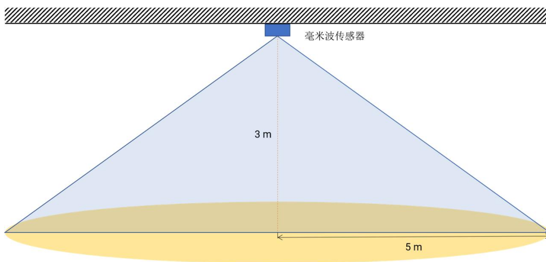
图 6-2 HLK-LD2402-L 挂顶安装检测范围示意图
