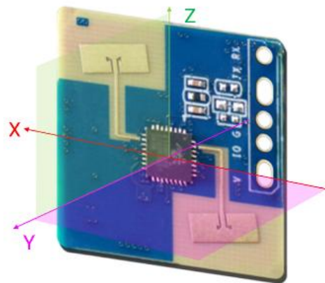
图 6-1 HLK-LD2402-L 方向定义示意图
