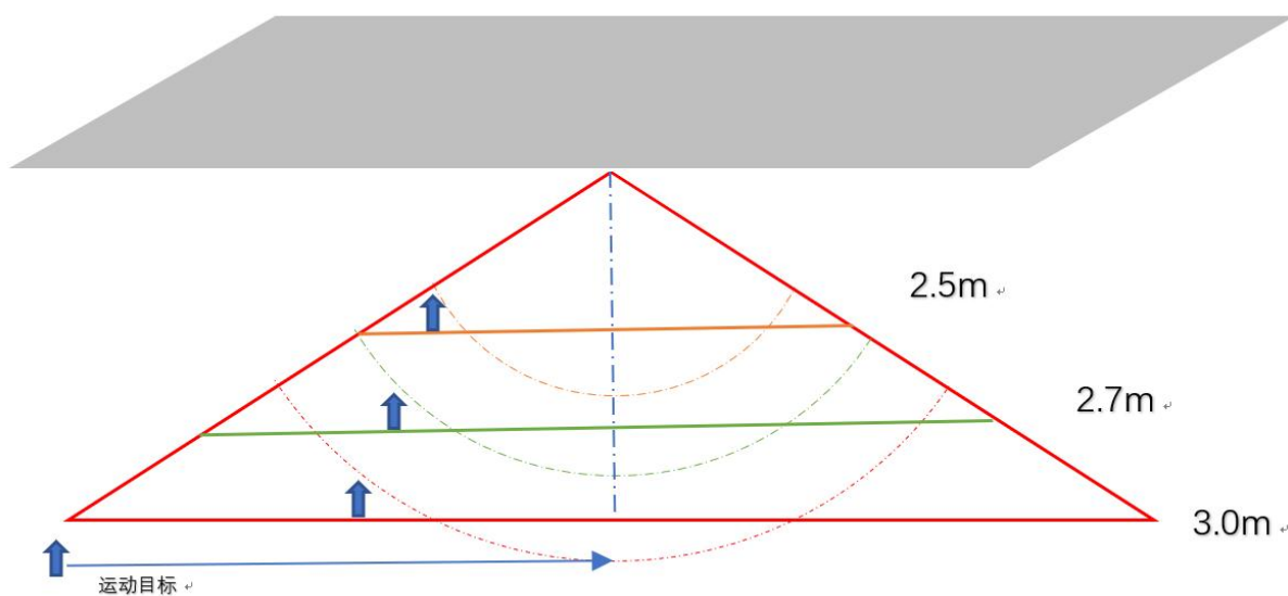
图 6-3 HLK-LD2402-L 挂顶安装高度与检测范围关系示意图
