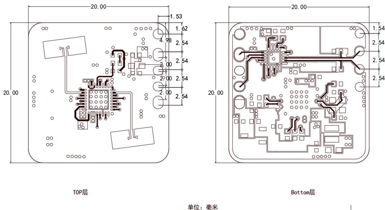
图 7-1 硬件 HLK-LD2402-L 机械尺寸
