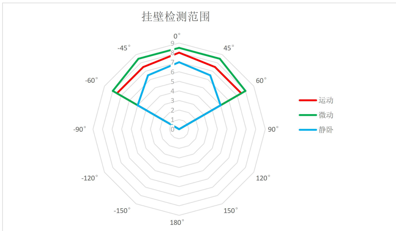
图 6-6 HLK-LD2402-L 挂壁安装感应范围
