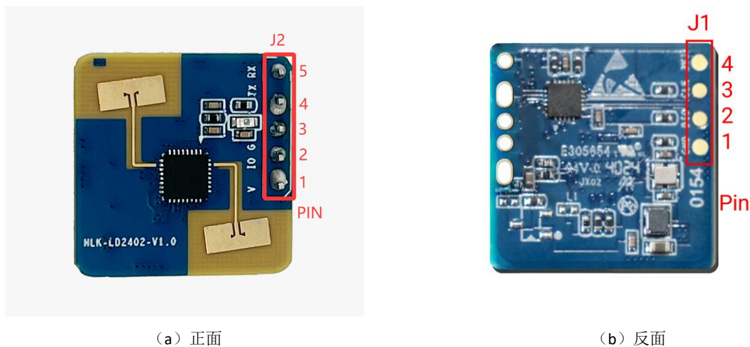
图 3-1 硬件 HLK-LD2402-L 正面与反面实物图
