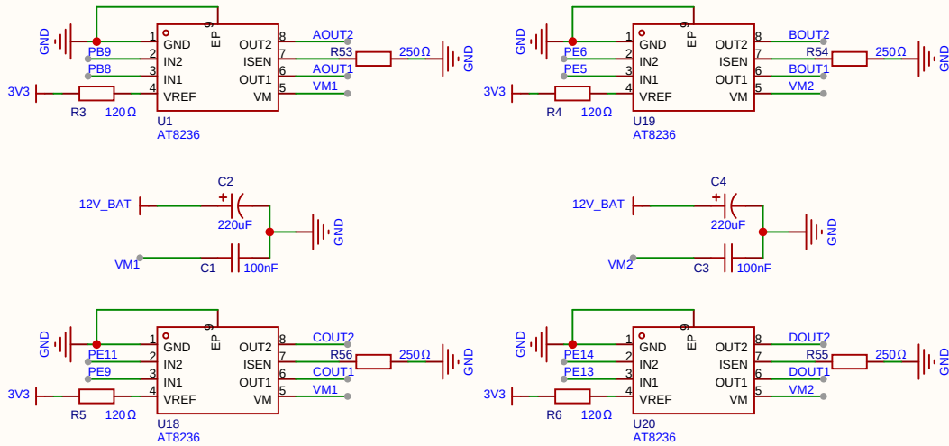
有刷电机驱动
