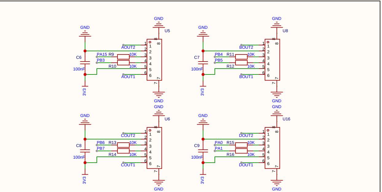
4路电机编码器接口
