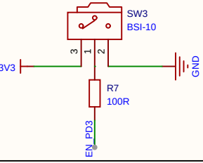
使能开关
