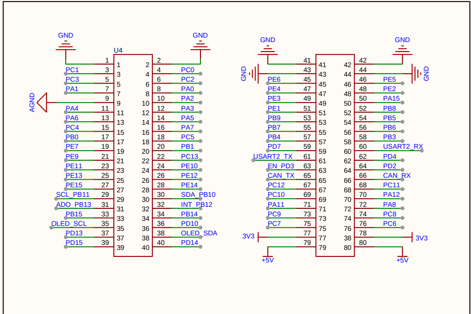
核心板接口
