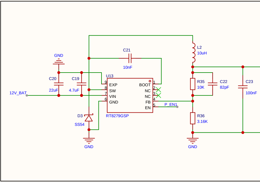
热控制电路
