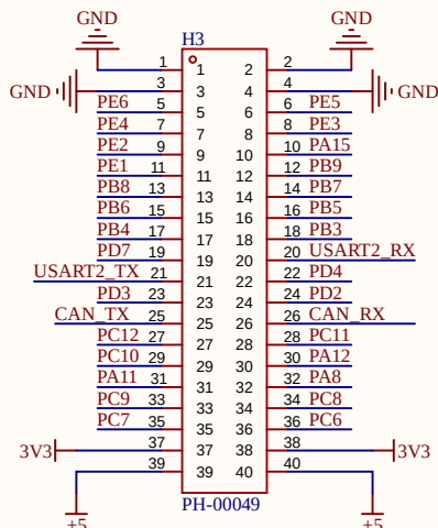
IO输入输出接口
