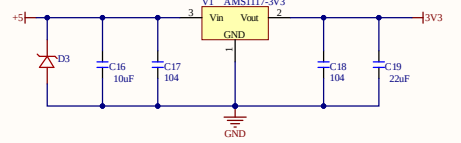
单片机电源
