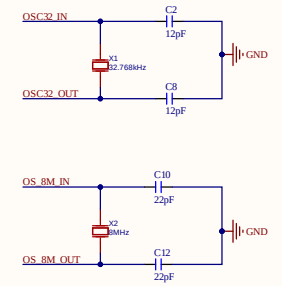
晶振电路
