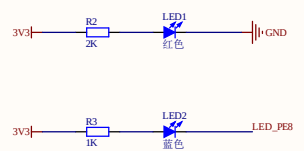
LED电路
