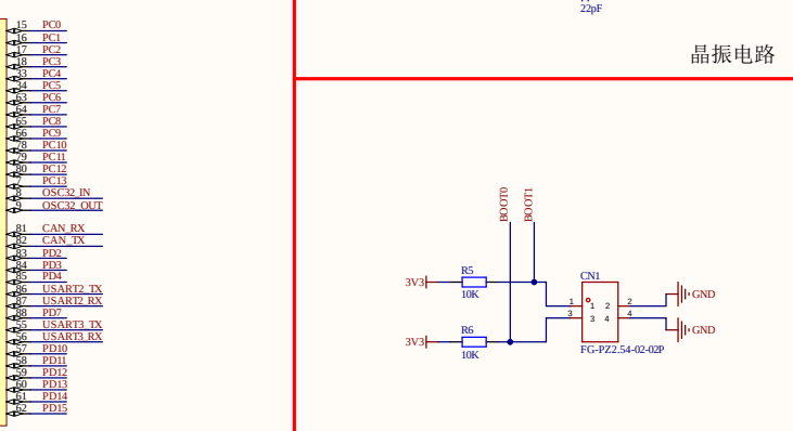
单片机主控
