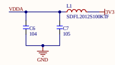
模拟电源
