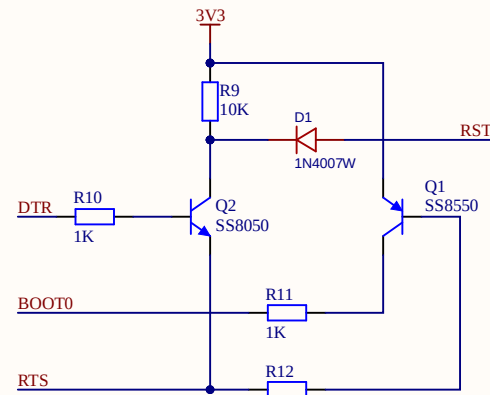
串口1一键下载电路
