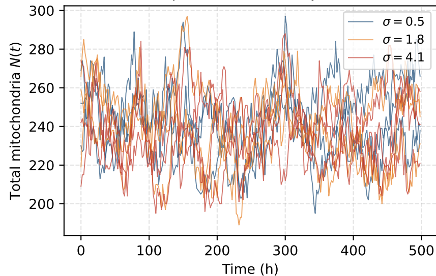
(d) Representative SSA trajectories
