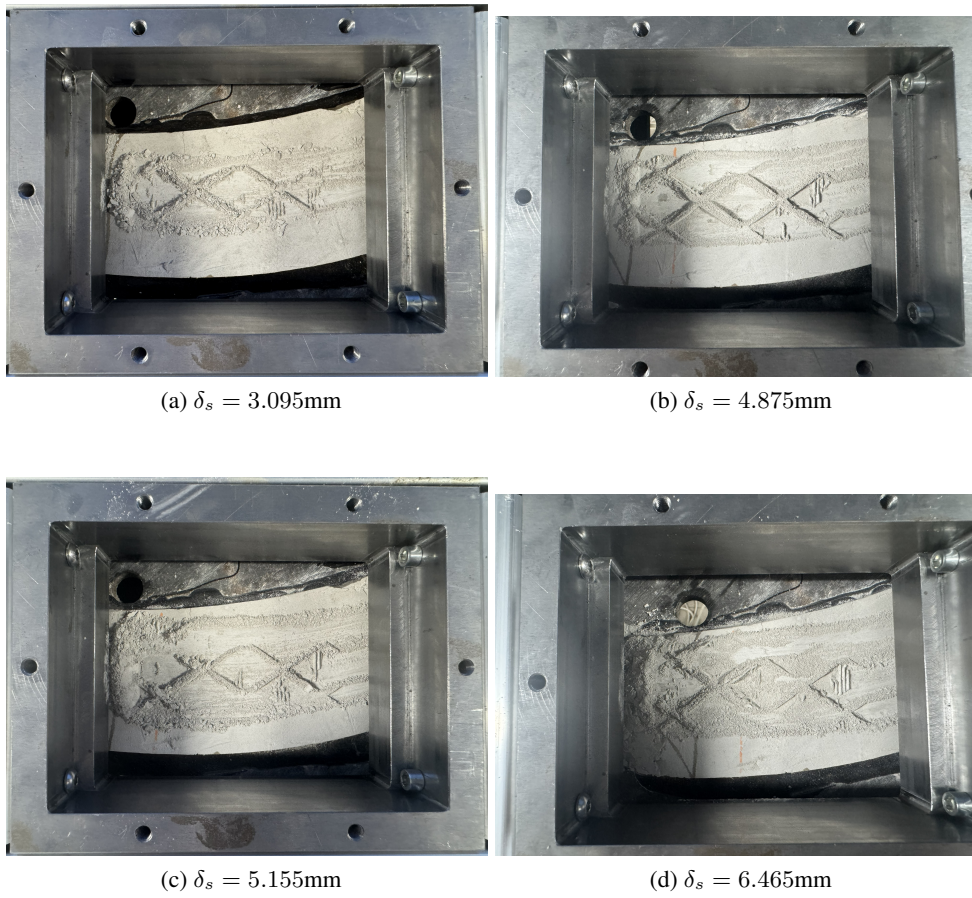
图 3.2: 垢层经刮削后的表面形貌 (不同弹簧压缩量)
