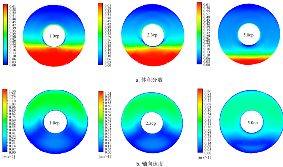
图 1.12: b 点不同洗井液粘度下砂砾体积分数和轴向速度云图
