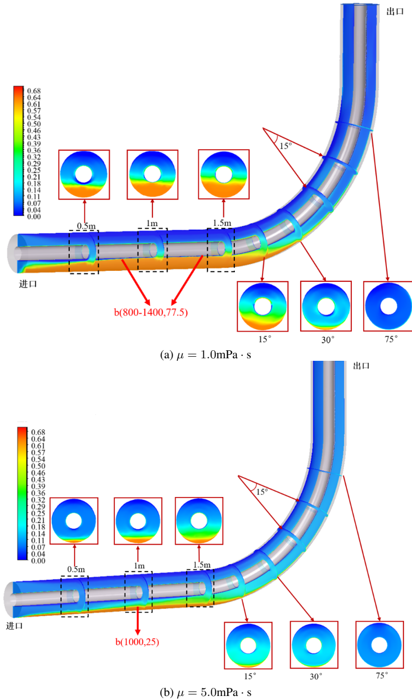
图 1.10: 不同粘度下环空内砂砾的体积分数云图
