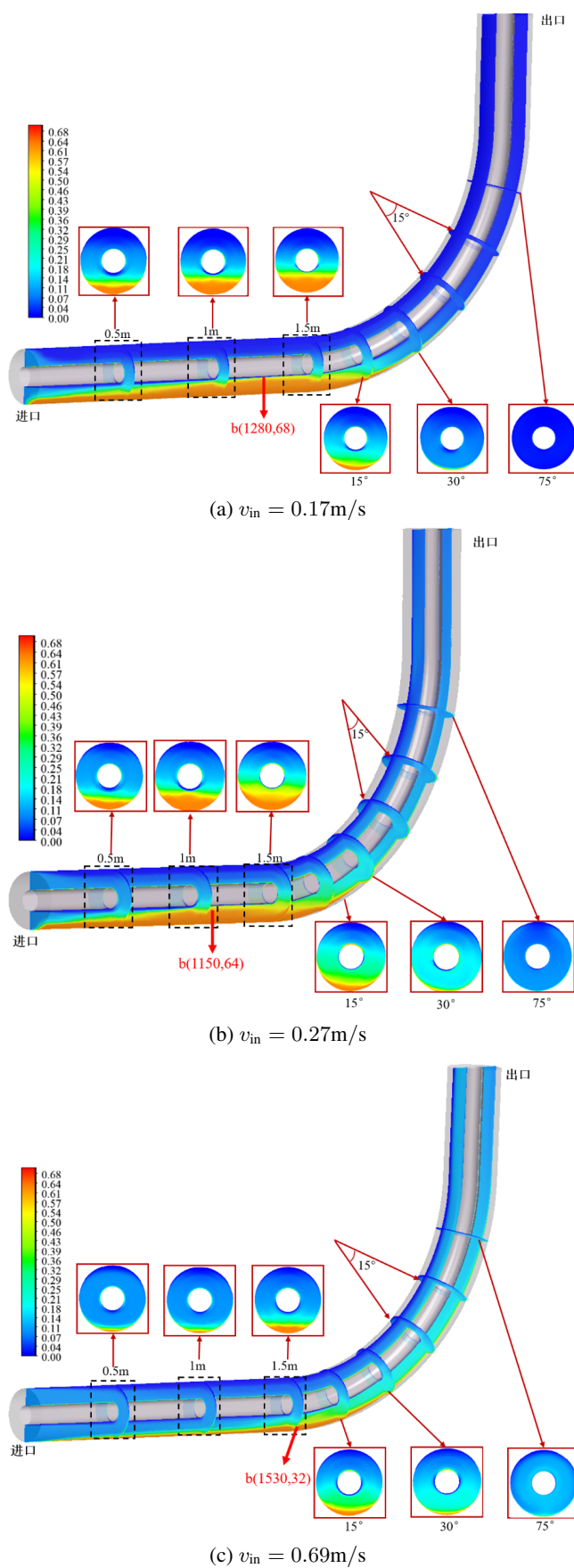
图 1.6: 流速对环空内砂砾的体积分数的影响
