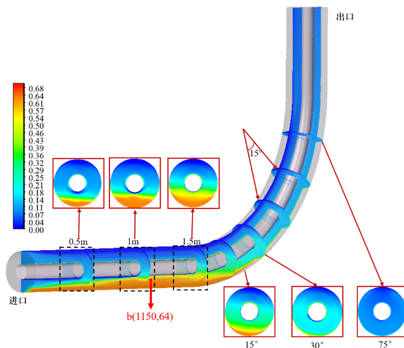
图 1.14: 流速为 0.27 m/s 时环空内砂砾的体积分数云图
