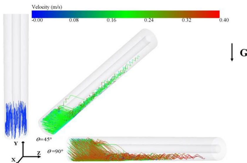
图 1.31: 井斜角对铁屑运动轨迹的影响
