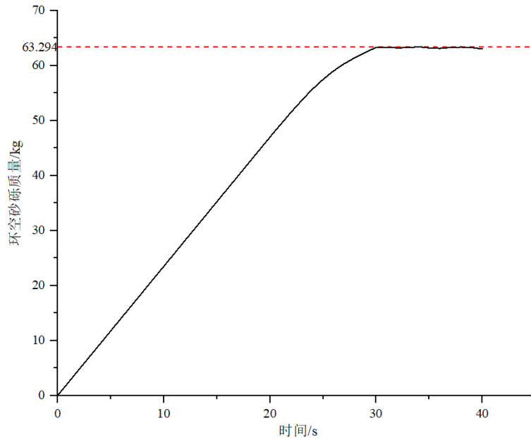
图 1.9: 环空内砂砾质量变化曲线
