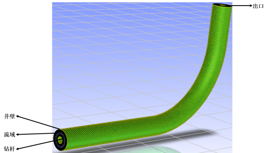
图 1.8: 环空三维模型
