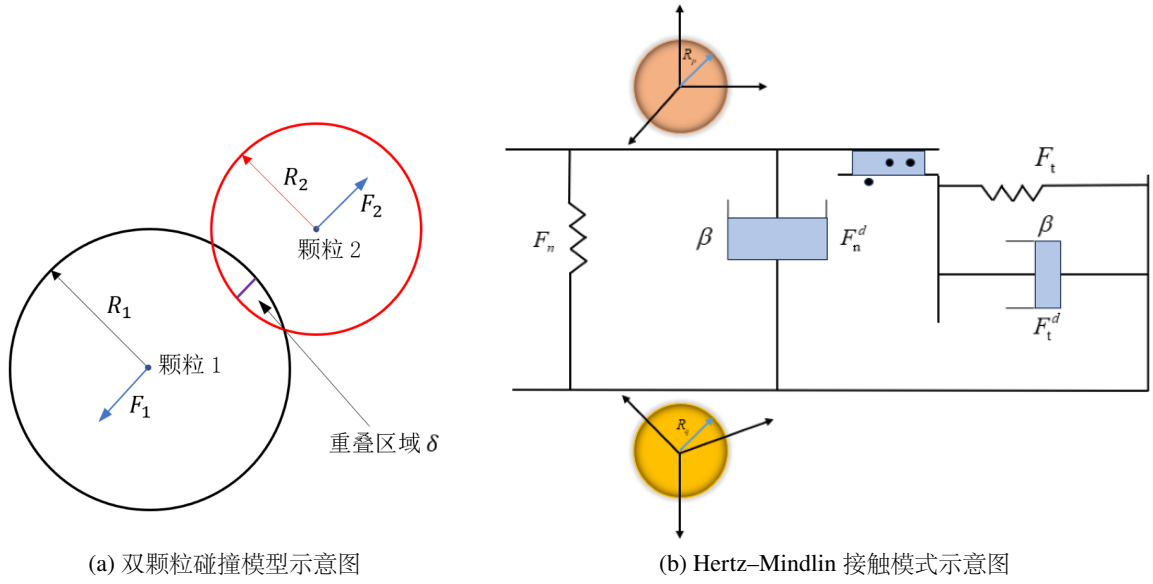
图 1.2: 颗粒-颗粒碰撞建模
