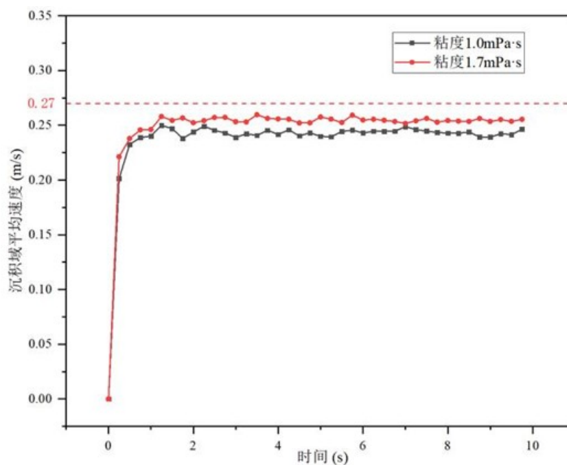
图 1.26: 洗井液粘度对铁屑颗粒运移速度时间演变的影响 ( \theta = 90^\circ , v_{\text{in}} = 0.27 \text{ m/s} )
