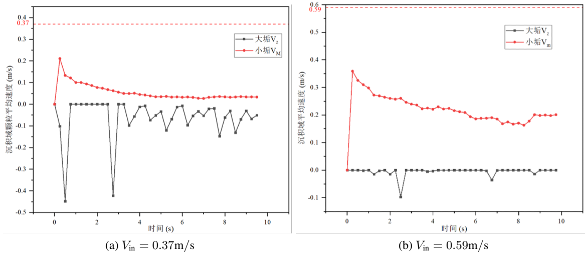
图 1.35: 钡锶垢颗粒在沉积域运移平均速度演化
