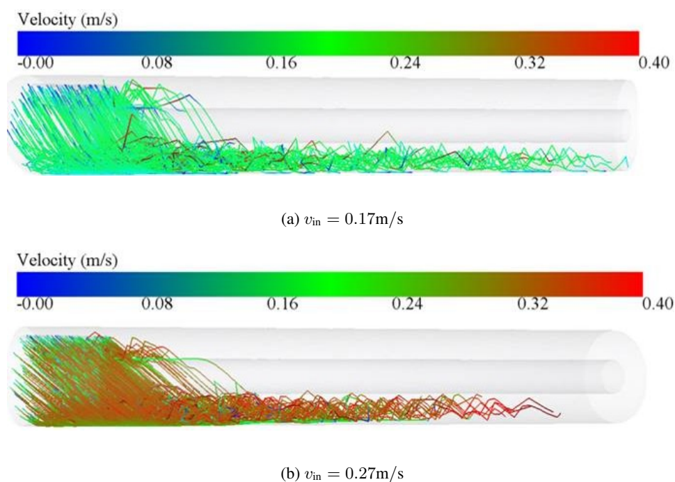
图 1.28: 洗井液流速对铁屑颗粒分布的影响 ( \theta = 90^\circ , \mu = 1.7\text{mPa} \cdot \text{s} )
