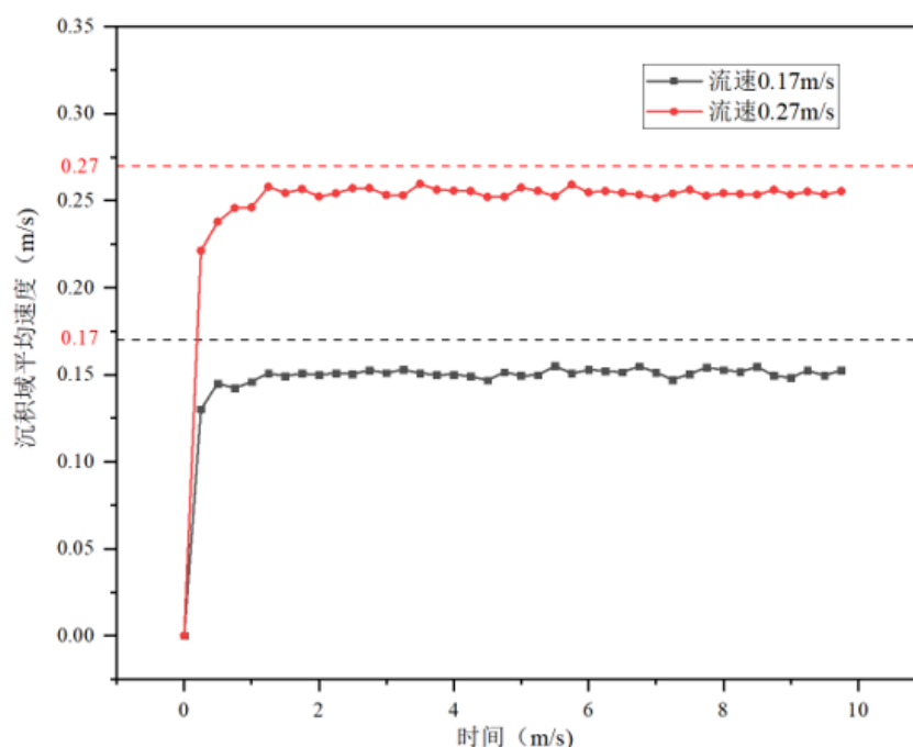
图 1.29: 洗井液速度对铁屑颗粒运移速度时间演变的影响 ( \mu = 1.7\text{mPa} \cdot \text{s} )
