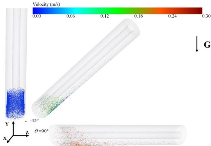
图 1.30: 井斜角对铁屑颗粒分布情况
