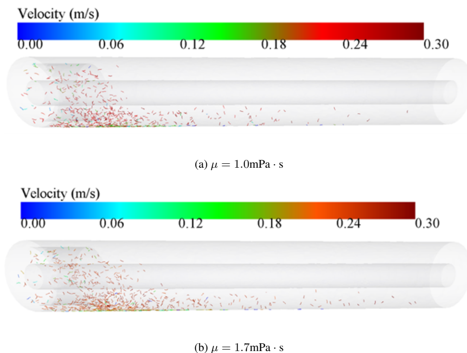
图 1.25: 洗井液粘度对铁屑颗粒速度分布的影响 ( \theta = 90^\circ , v_{\text{in}} = 0.27 \text{ m/s} )
