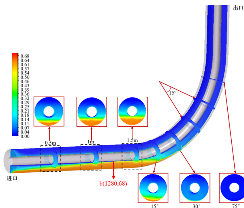
图 1.13: 流速为 0.17 m/s 时环空内砂砾的体积分数云图
