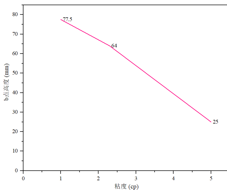
图 1.21: b 点高度随洗井液粘度变化曲线
