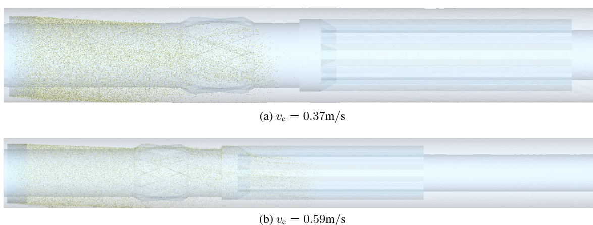
图 1.7: 相同时间步不同环空流速下砂砾颗粒分布
