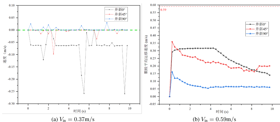
图 1.37: 钡锶垢颗粒在沉积域运移平均速度演化
