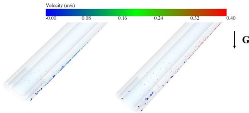
图 1.34: 钡锬垢颗粒在井筒中的运移
