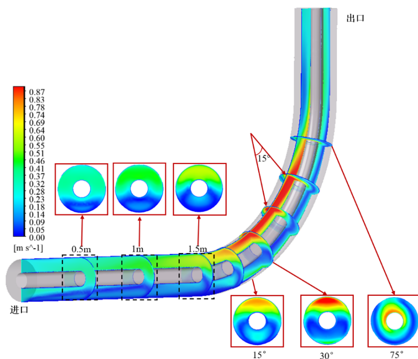
图 1.10: 不同截面砂砾速度云图
