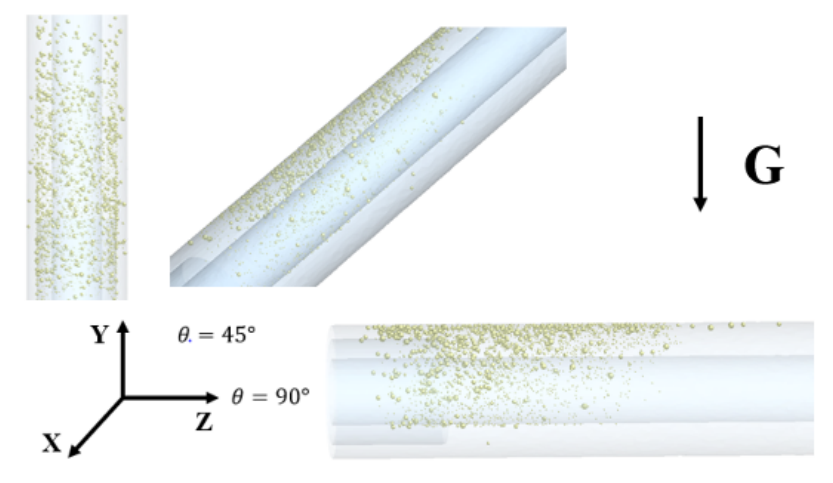
图 1.39: 不同井斜下蜡垢颗粒井筒内运移分布图
