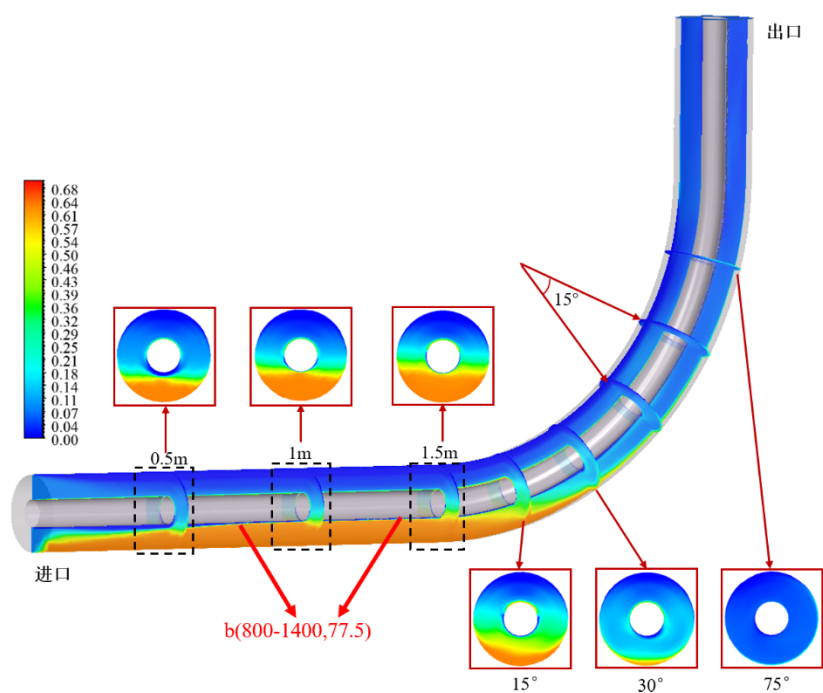
图 1.19: 粘度为 1.0 cp 时环空内砂砾的体积分数云图
