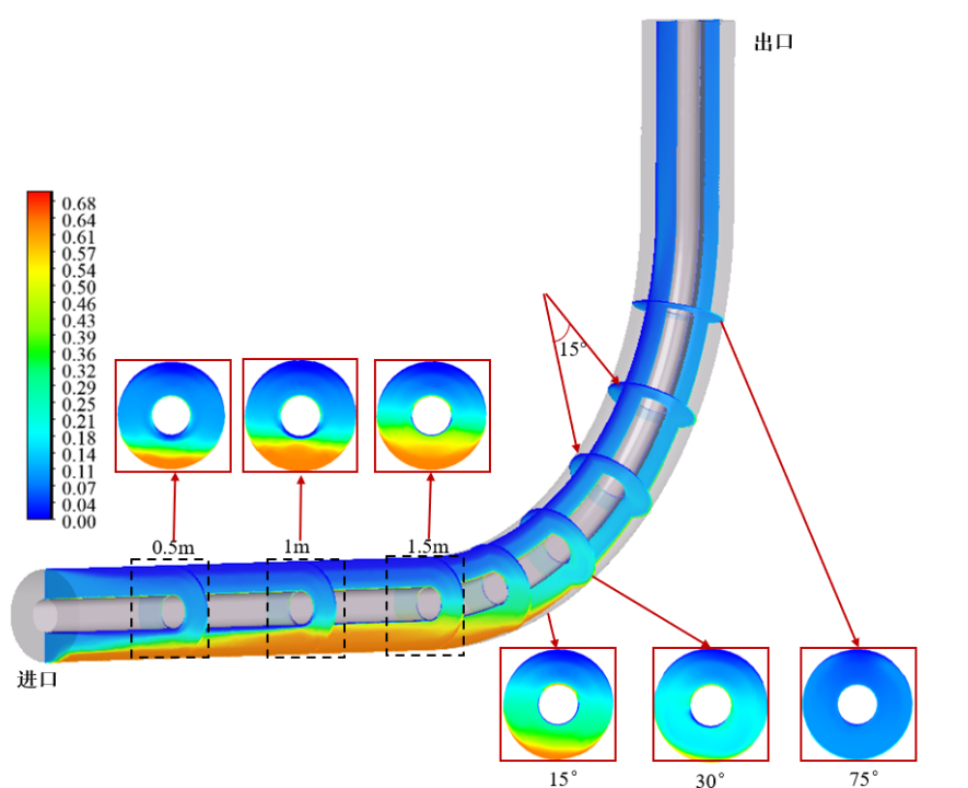
图 1.11: 不同截面砂砾体积分数云图
