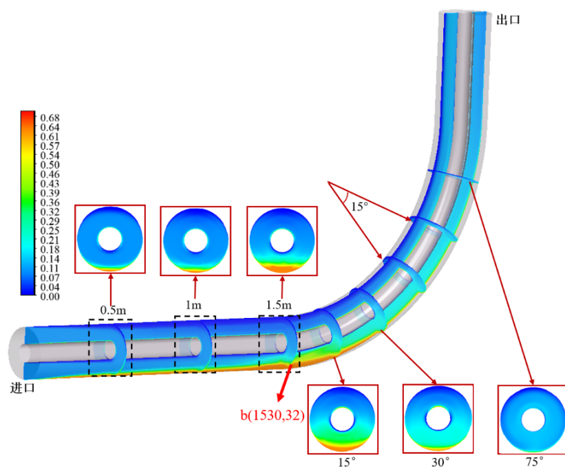
图 1.15: 流速为 0.69 m/s 时环空内砂砾的体积分数云图
