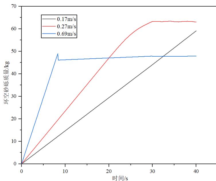
图 1.12: 不同流速下环空内砂砾质量随时间的变化曲线
