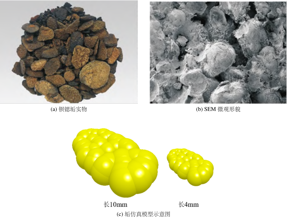
图 1.33: 钡锶垢颗粒及仿真模型对比
