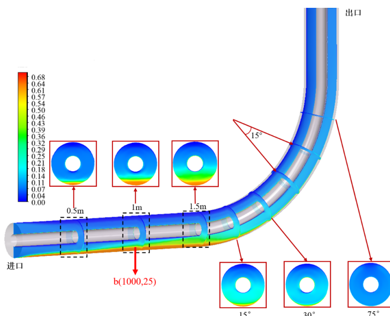
图 1.20: 粘度为 5.0 cp 时环空内砂砾的体积分数云图
