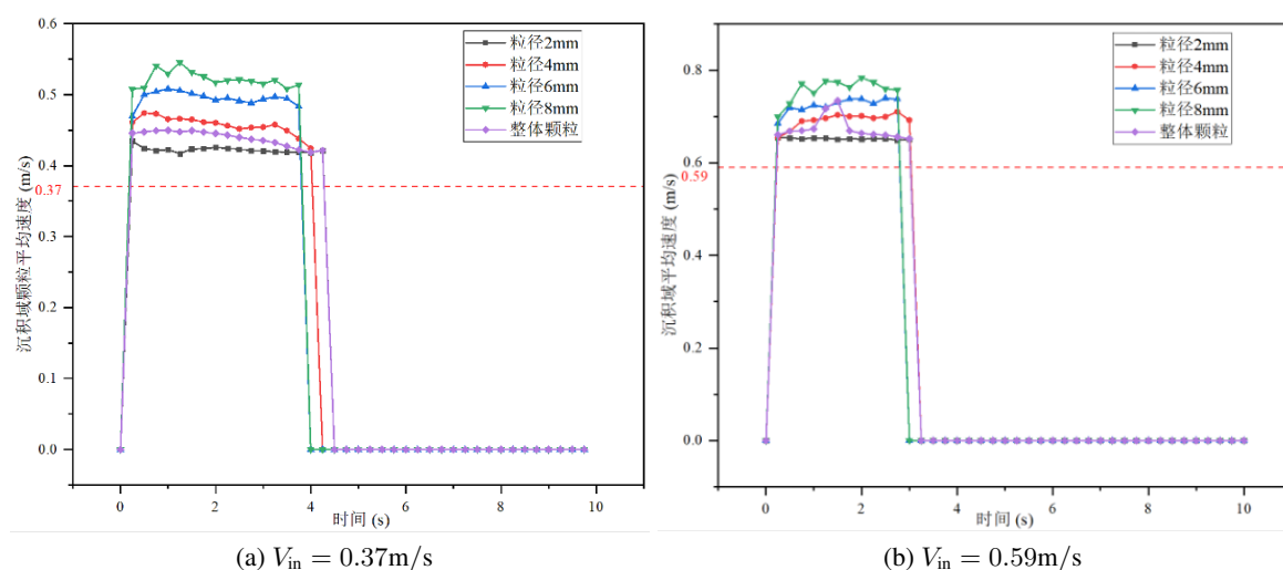
图 1.38: 蜡垢颗粒在沉积域运移平均速度演化
