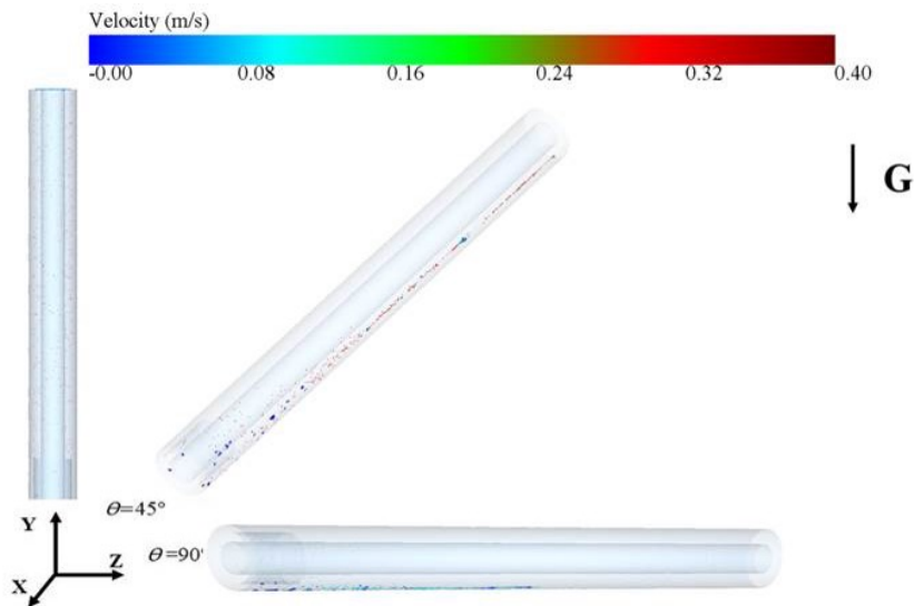
图 1.36: 钡锶垢颗粒在井筒中的运移
