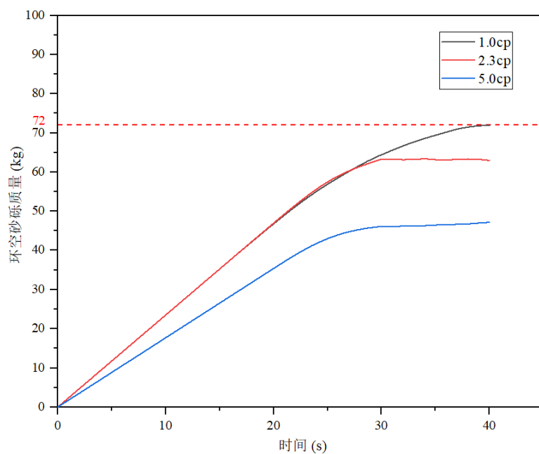
图 1.18: 不同粘度下环空内砂砾质量随时间的变化曲线
