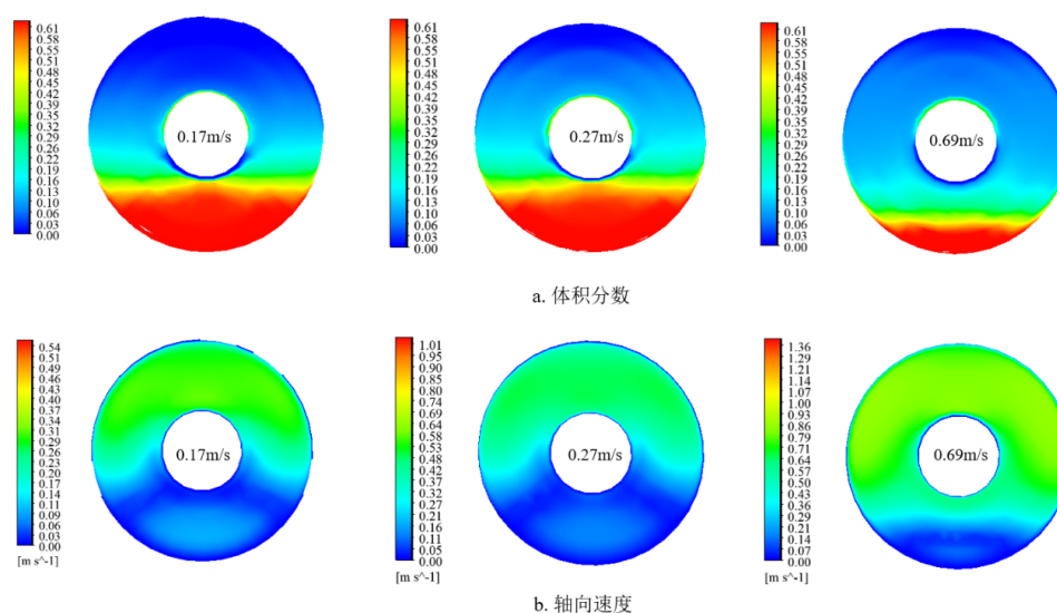
图 1.17: b 点不同洗井液流速下砂砾体积分数和轴向速度云图
