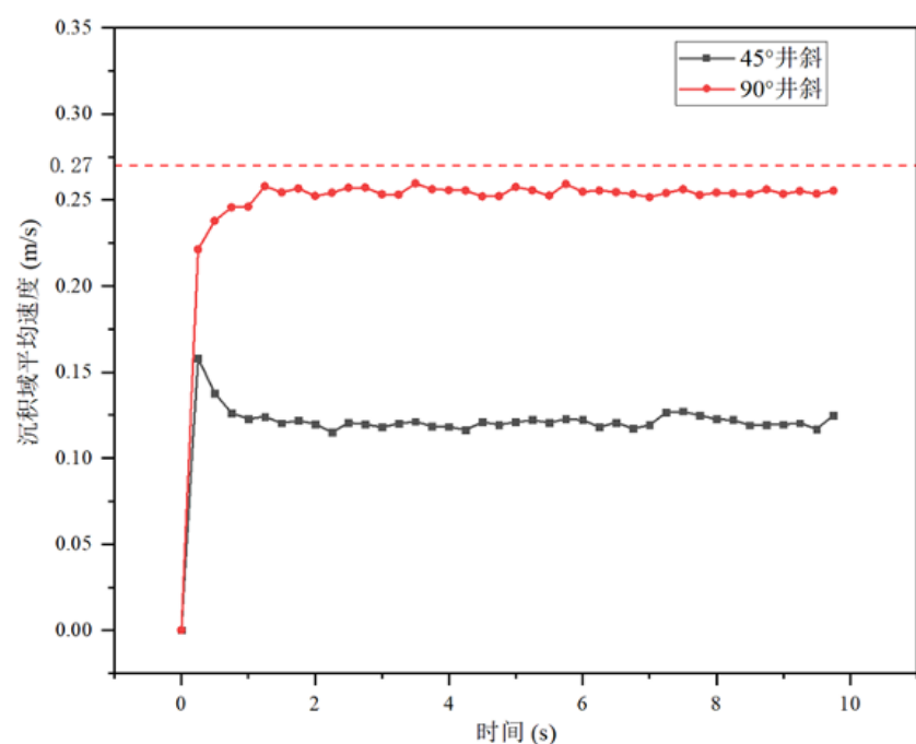
图 1.32: 井斜角对铁屑运动速度的影响
