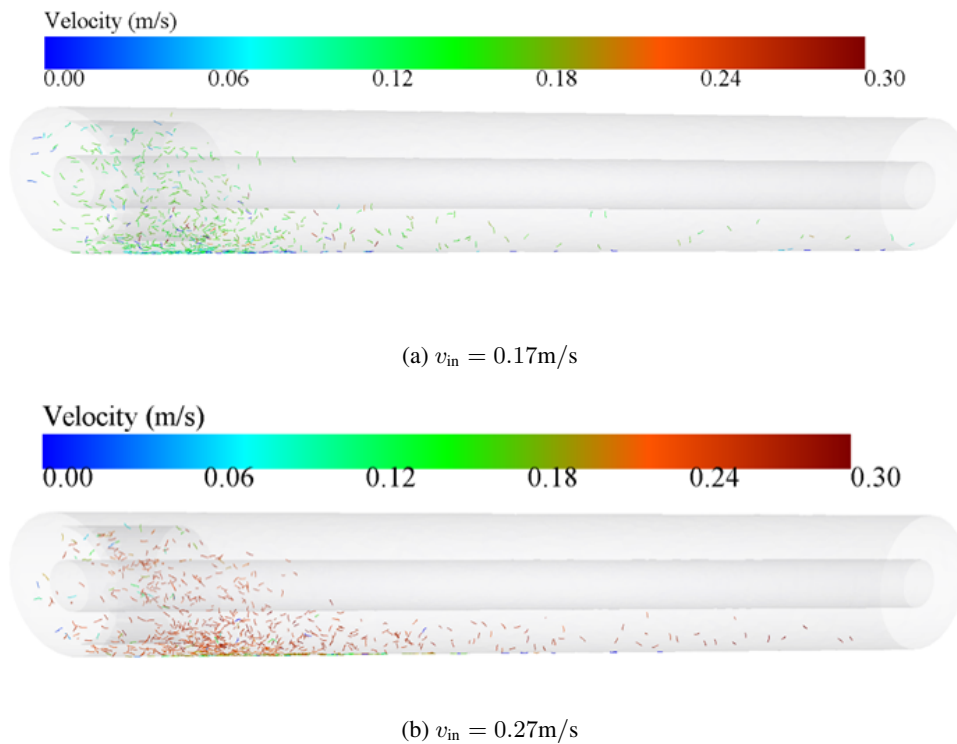
图 1.27: 洗井液流速对铁屑颗粒分布的影响 ( \theta = 90^\circ , \mu = 1.7\text{mPa} \cdot \text{s} )
