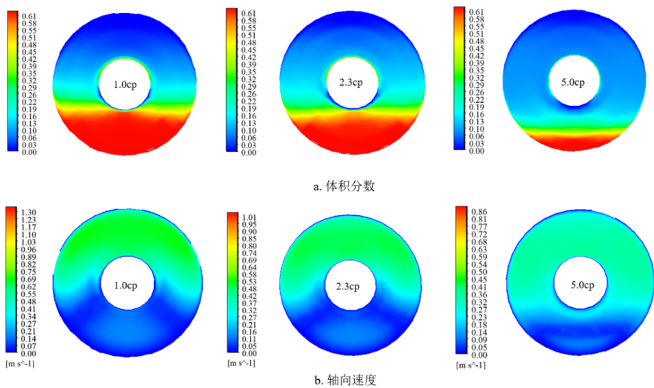
图 1.22: b 点不同洗井液粘度下砂砾体积分数和轴向速度云图
