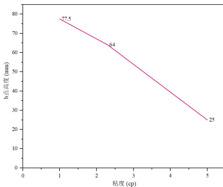
图 1.22: b 点高度随洗井液粘度变化曲线
