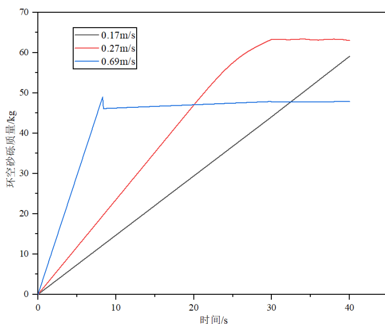
图 1.13: 不同流速下环空内砂砾质量随时间的变化曲线
