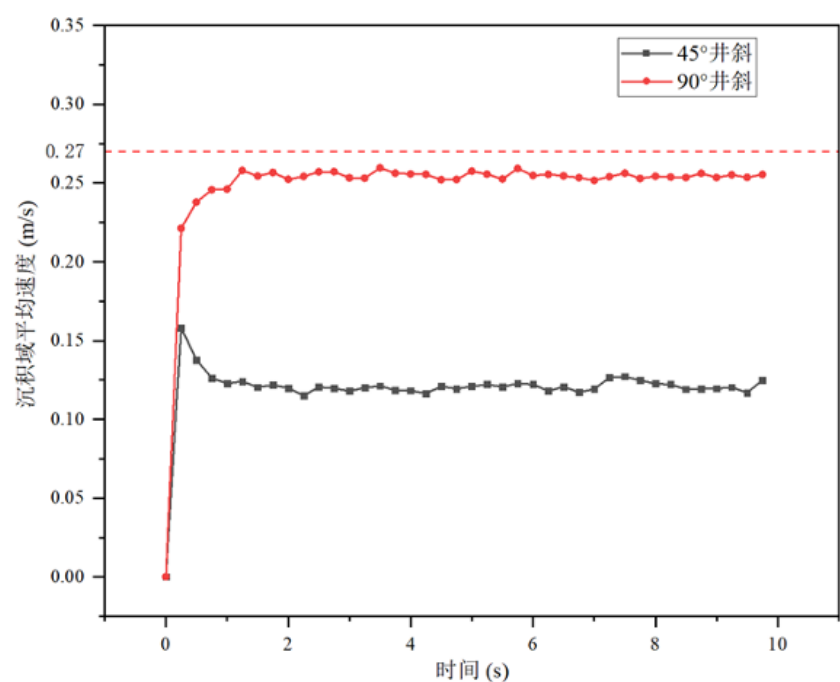
图 1.33: 井斜角对铁屑运动速度的影响
