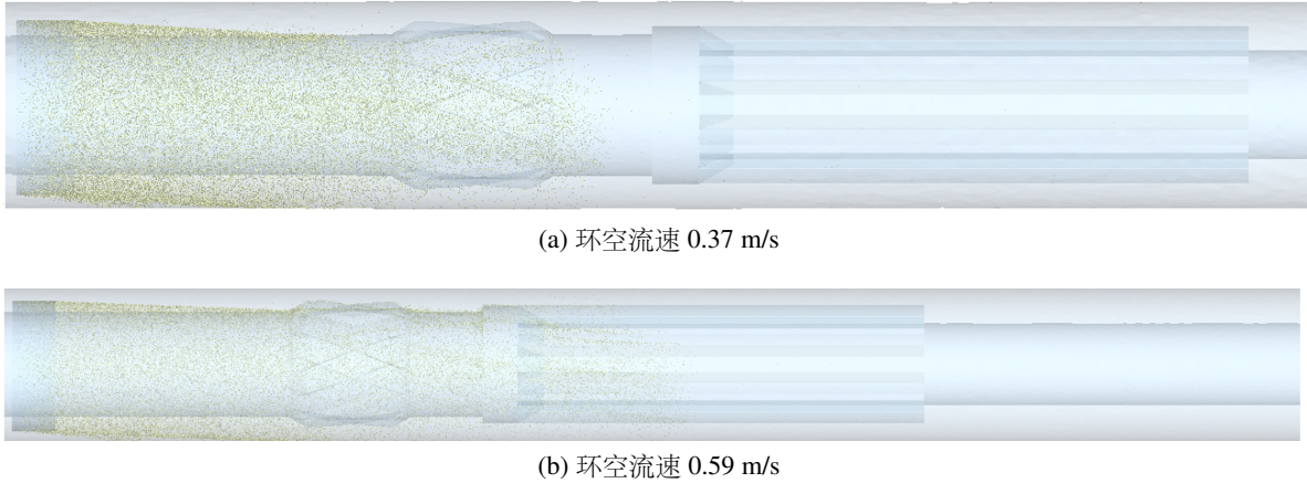
图 1.8: 相同时间步不同环空流速下砂砾颗粒分布
