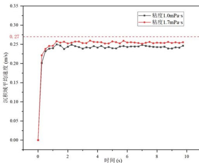
图 1.27: 洗井液粘度对铁屑颗粒运移速度时间演变的影响 ( \theta = 90^\circ , v_{in} = 0.27\text{m/s} )
