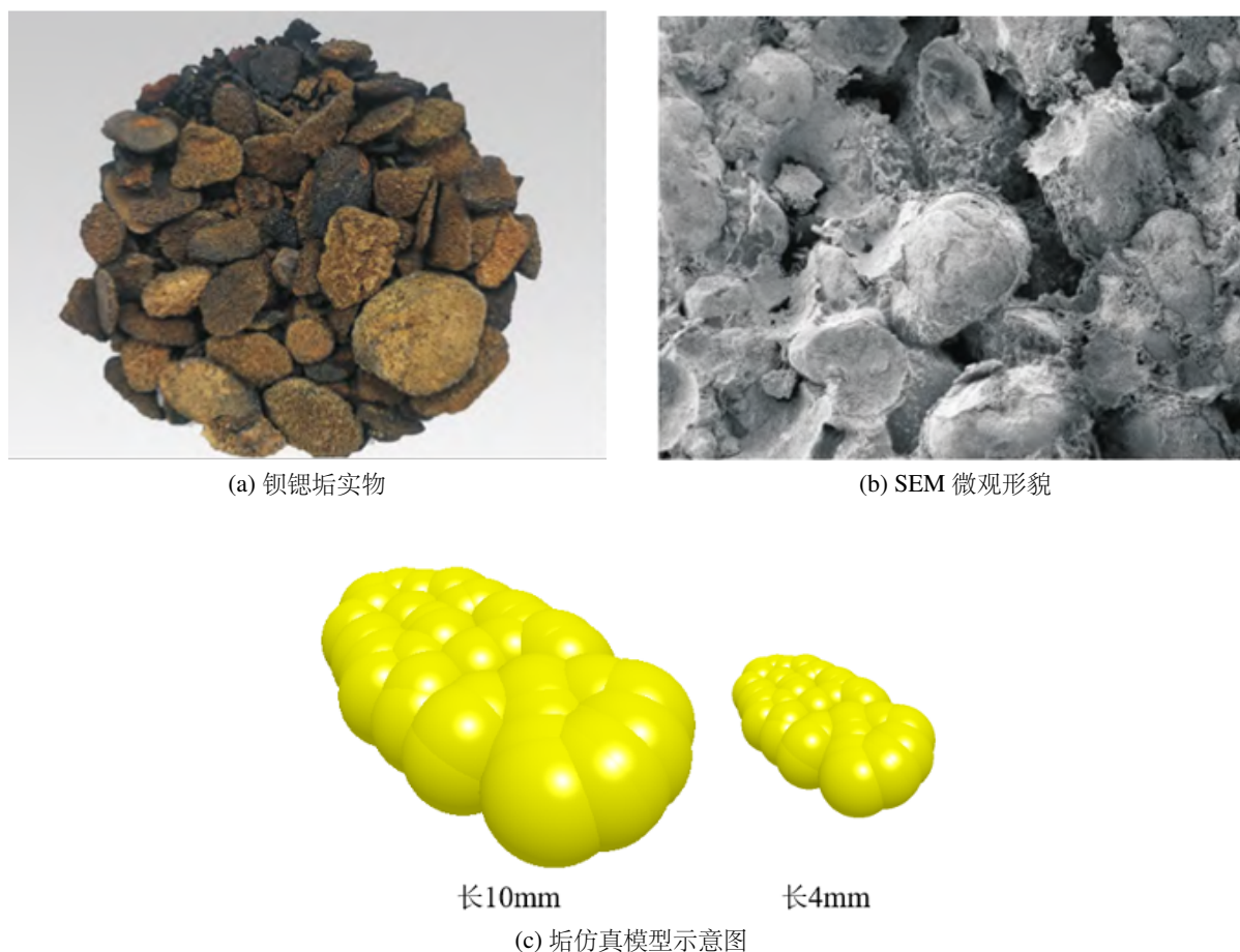
图 1.34: 钡锶垢颗粒及仿真模型对比
