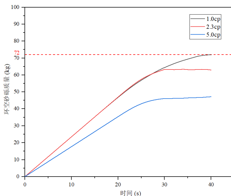
图 1.19: 不同粘度下环空内砂砾质量随时间的变化曲线
