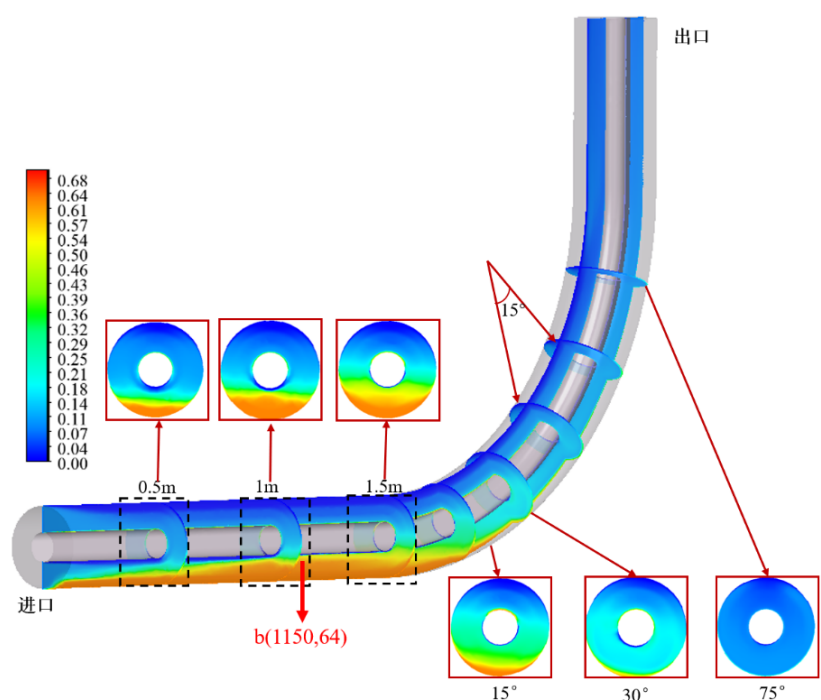
图 1.15: 流速为 0.27 m/s 时环空内砂砾的体积分数云图
