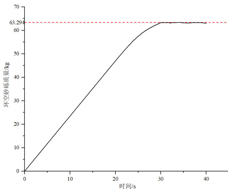
图 1.10: 环空内砂砾质量变化曲线
