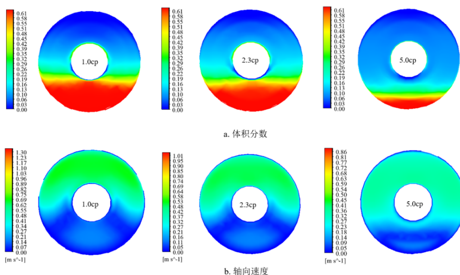
图 1.23: b 点不同洗井液粘度下砂砾体积分数和轴向速度云图
