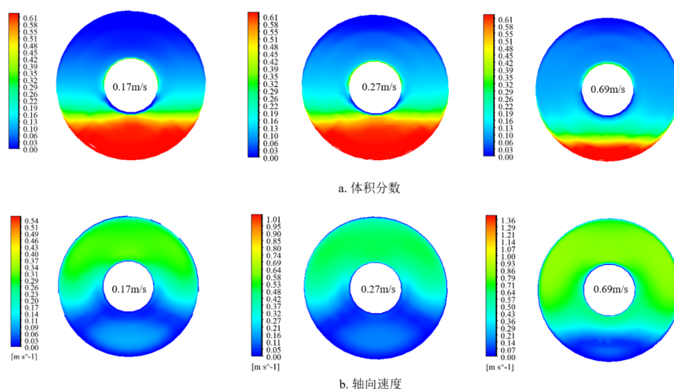
图 1.18: b 点不同洗井液流速下砂砾体积分数和轴向速度云图
