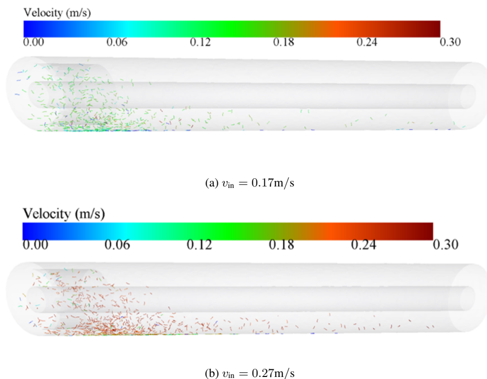
图 1.28: 洗井液流速对铁屑颗粒分布的影响 ( \theta = 90^\circ , \mu = 1.7\text{mPa} \cdot \text{s} )
