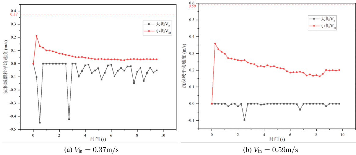
图 1.36: 钡锶垢颗粒在沉积域运移平均速度演化
