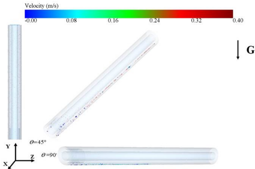
图 1.37: 钡锶垢颗粒在井筒中的运移
