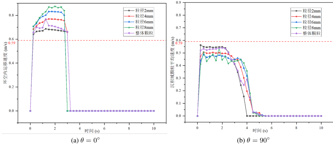
图 1.41: 井斜对蜡垢颗粒在沉积域运移平均速度演化的影响
