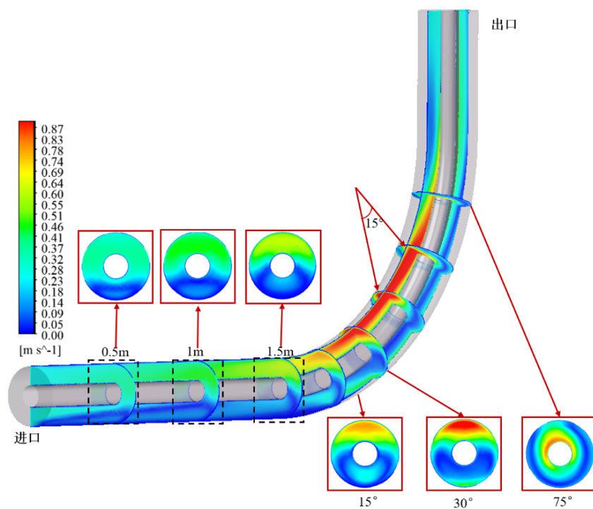
图 1.11: 不同截面砂砾速度云图
