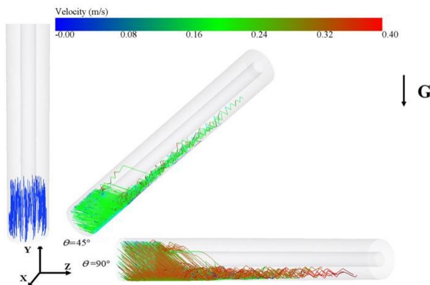
图 1.32: 井斜角对铁屑运动轨迹的影响
