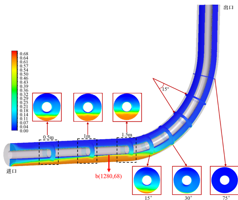
图 1.14: 流速为 0.17 m/s 时环空内砂砾的体积分数云图
