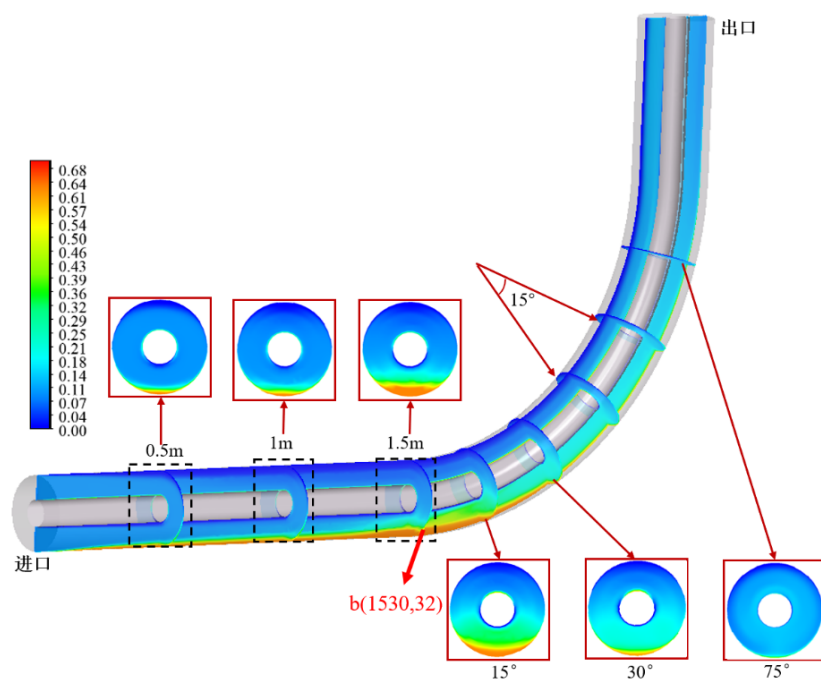
图 1.16: 流速为 0.69 m/s 时环空内砂砾的体积分数云图
