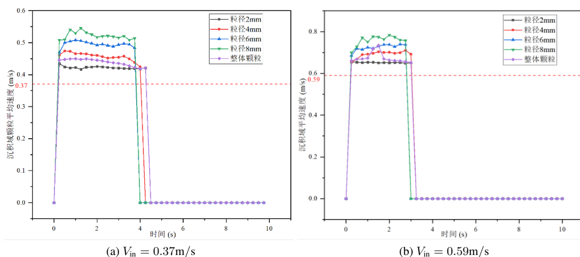
图 1.39: 蜡垢颗粒在沉积域运移平均速度演化
