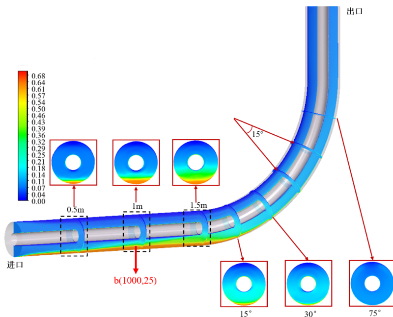
图 1.21: 粘度为 5.0 cp 时环空内砂砾的体积分数云图
