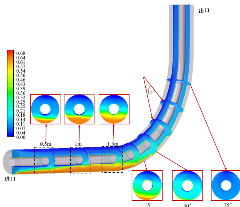
图 1.12: 不同截面砂砾体积分数云图
