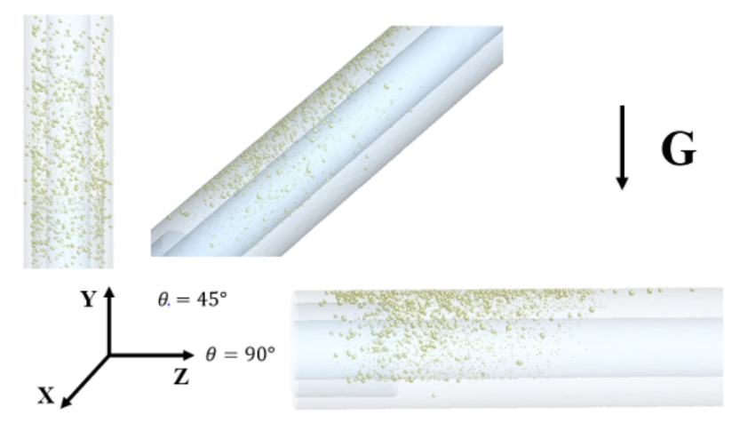
图 1.40: 不同井斜下蜡垢颗粒井筒内运移分布图
