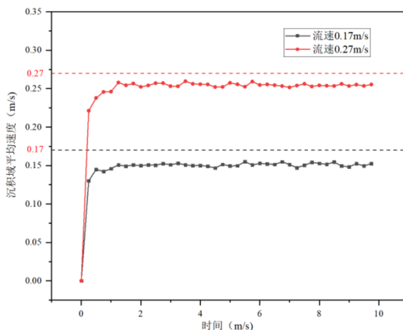
图 1.30: 洗井液速度对铁屑颗粒运移速度时间演变的影响 ( \mu = 1.7\text{mPa} \cdot \text{s} )
