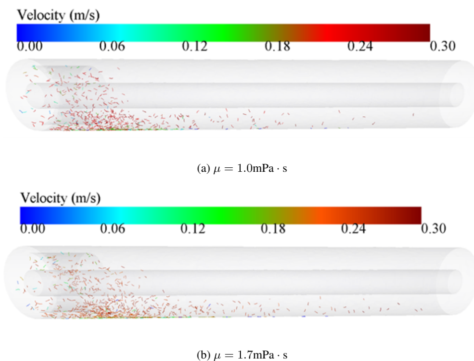
图 1.26: 洗井液粘度对铁屑颗粒速度分布的影响 ( \theta = 90^\circ , v_{in} = 0.27 \text{ m/s} )
