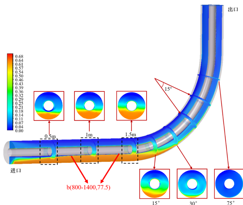
图 1.20: 粘度为 1.0 cp 时环空内砂砾的体积分数云图
