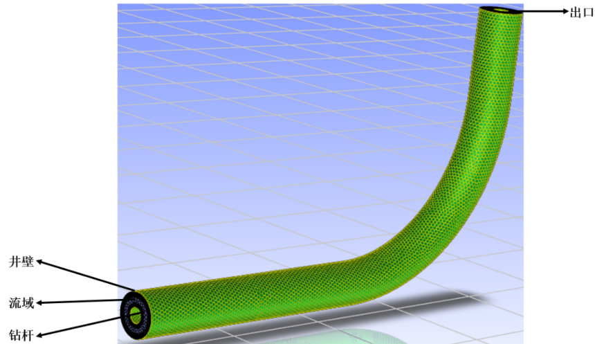
图 1.9: 环空三维模型
