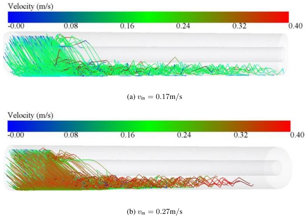
图 1.29: 洗井液流速对铁屑颗粒分布的影响 ( \theta = 90^\circ , \mu = 1.7\text{mPa} \cdot \text{s} )
