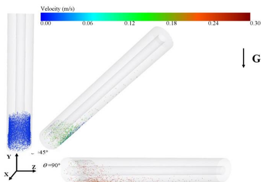
图 1.31: 井斜角对铁屑颗粒分布情况
