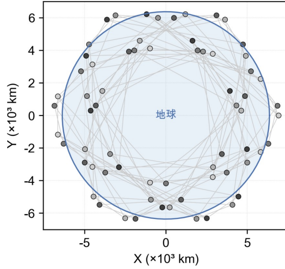
图 2 Walker Delta 星座与+Grid 链路拓扑示意
