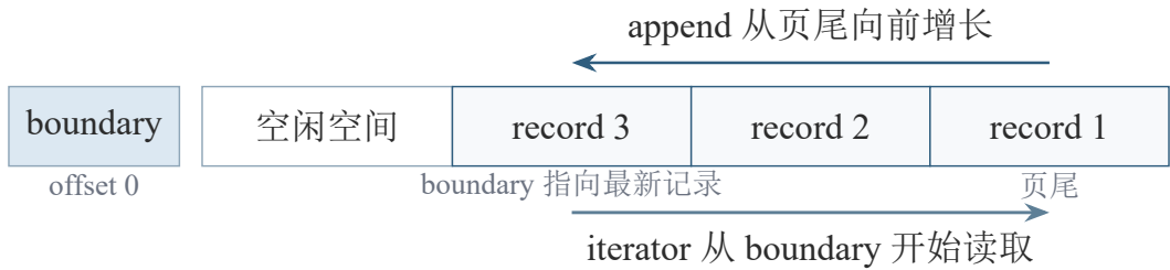
图 3-2 日志页内记录布局示意
