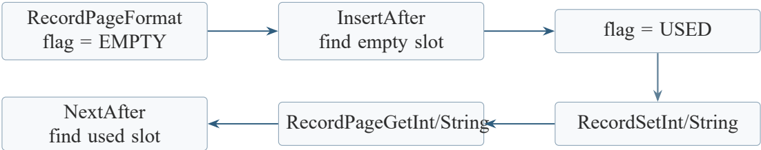
图 6-3 RecordPage 中一个记录槽的基本生命周期
